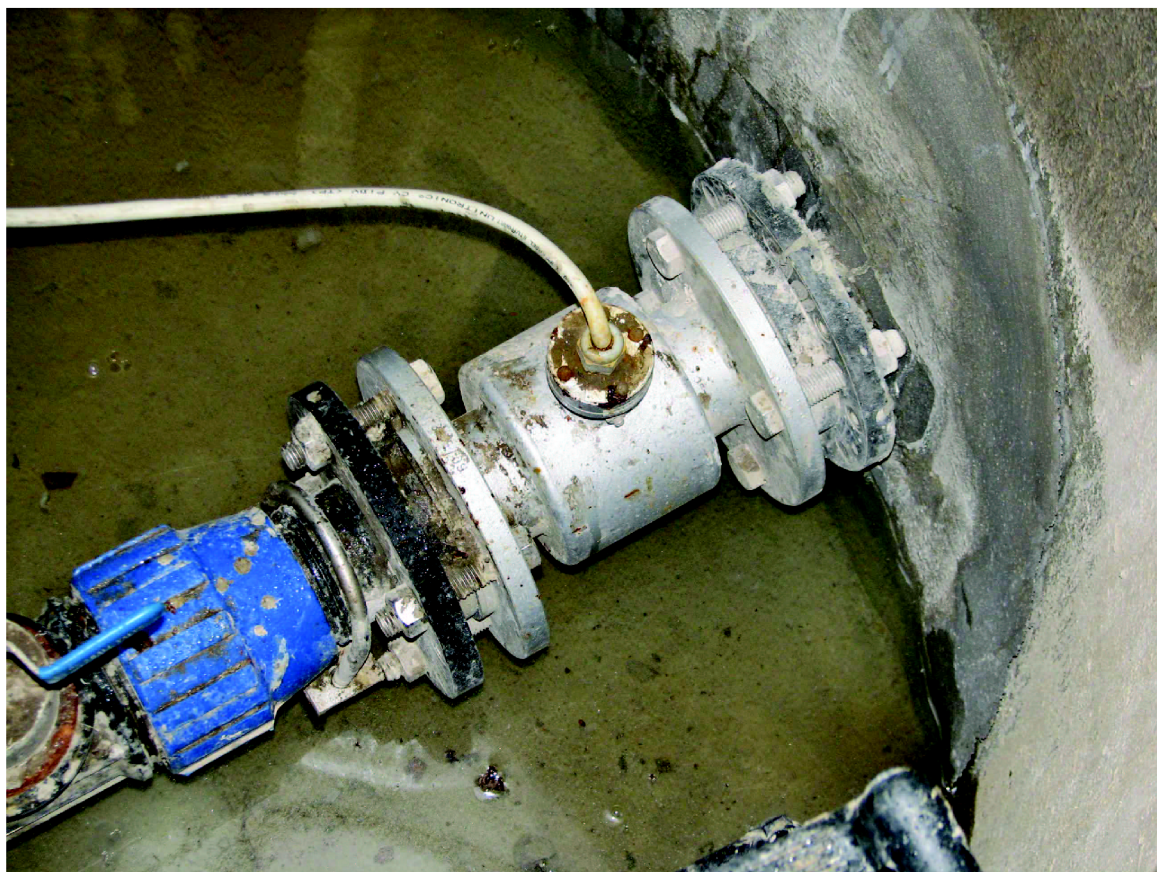
Obr. 3.9 Osazení indukčního průtokoměru v šachtě
