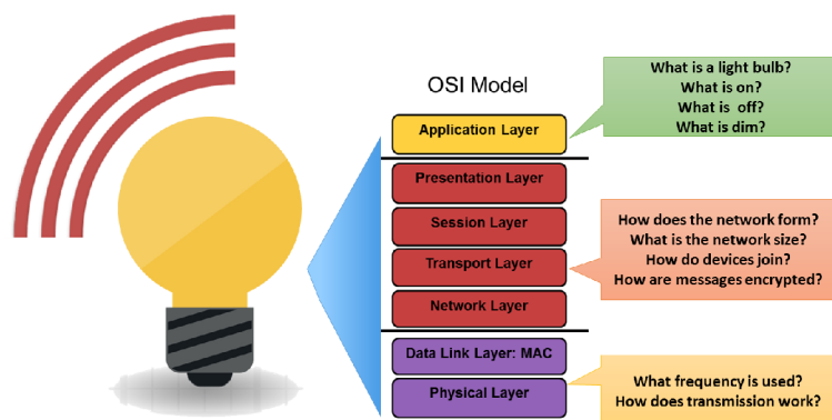
Obr. 3.1: Model ISO OSI aplikačného štandardu ZigBee [25]
