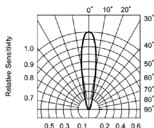
Obr. 8.2: Diagram senzitivity fototranzistoru
