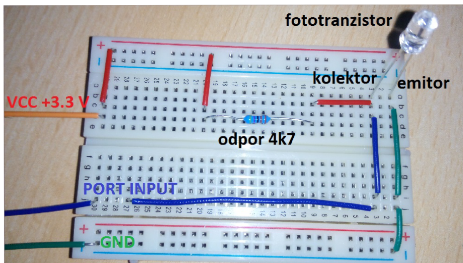
Obr. 8.4: Fyzická realizácia obvodu
