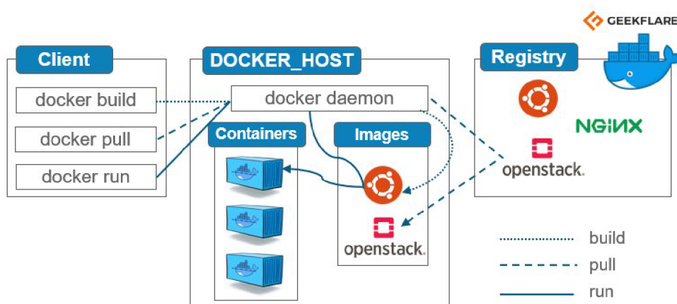
Obrázek 5: Architektura dockeru [8]
