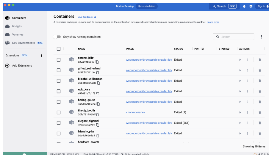
Obrázek 6: Docker GUI
