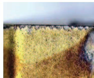
Vyštipování břitu
