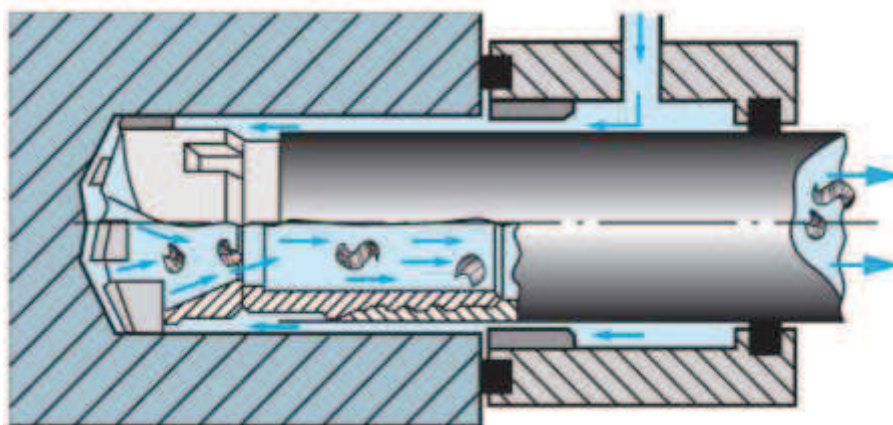
Obr. 13 Systém s jednou trubkou (STS) [37].
