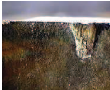
Vylamování ostří
