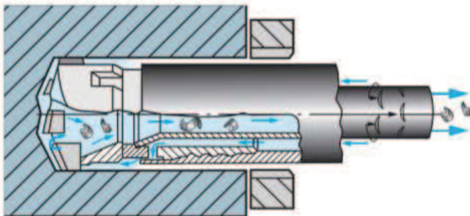
Obr. 12 Ejektorový systém [37].
