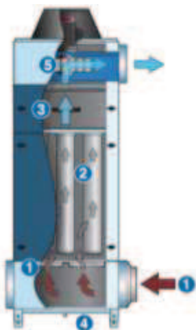
Obr. 25 Filtr olejové mlhy [26].
