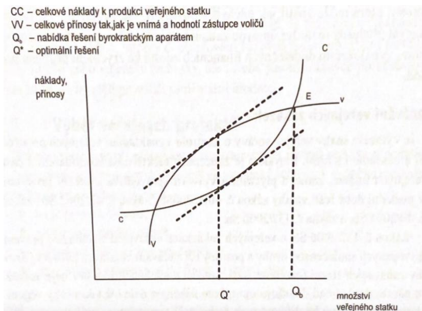
Obrázek 4 Niskanenův model
