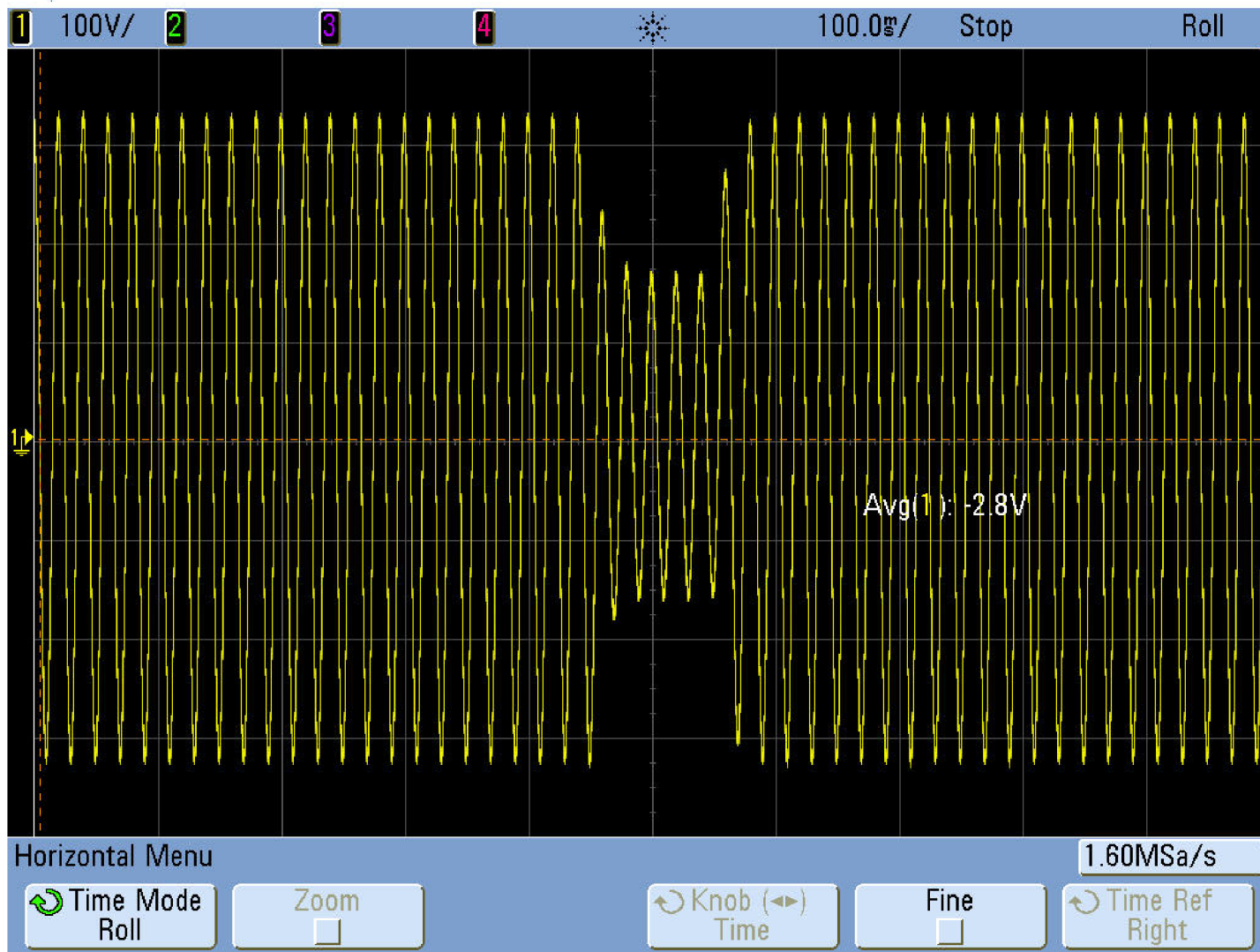
Obr. B.4: Zachycený pokles napětí osciloskopem Agilent.
