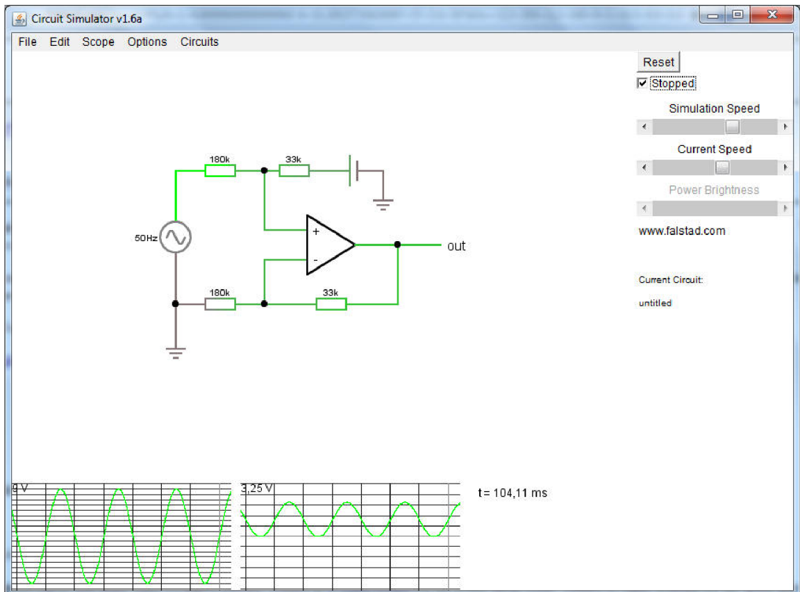
Obr. A.1: Simulace napěťového přenosu úrovnňového zesilovače.
