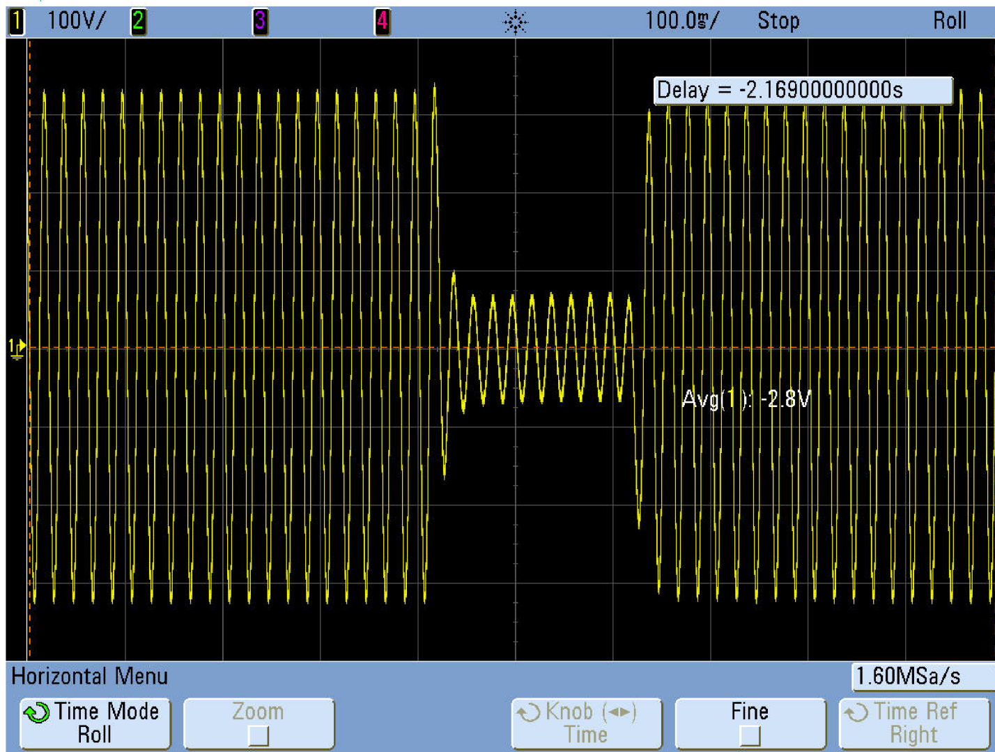
Obr. B.5: Zachycený pokles napětí osciloskopem Agilent.
