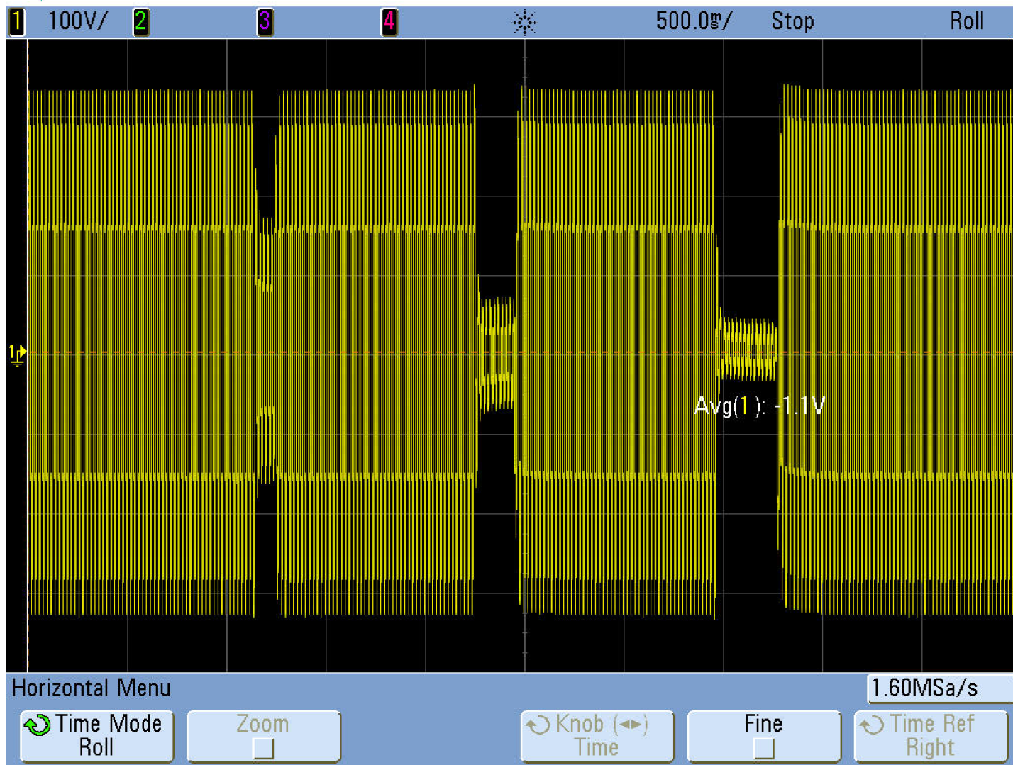
Obr. B.7: Zachycený pokles napětí osciloskopem Agilent.
