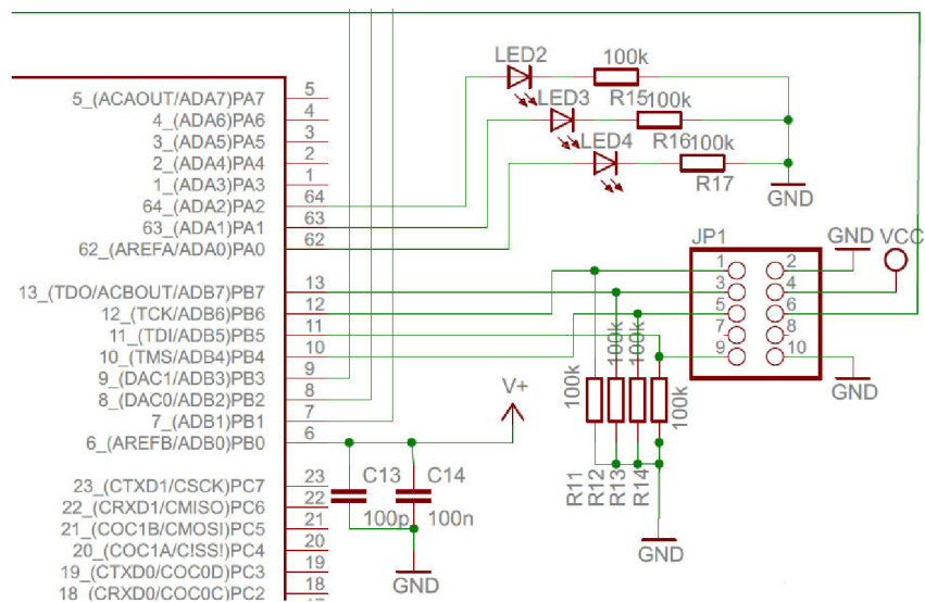
Obr. 3.4: Připojení rozhraní JTAG a indikačních diod k mikrokontroléru.
