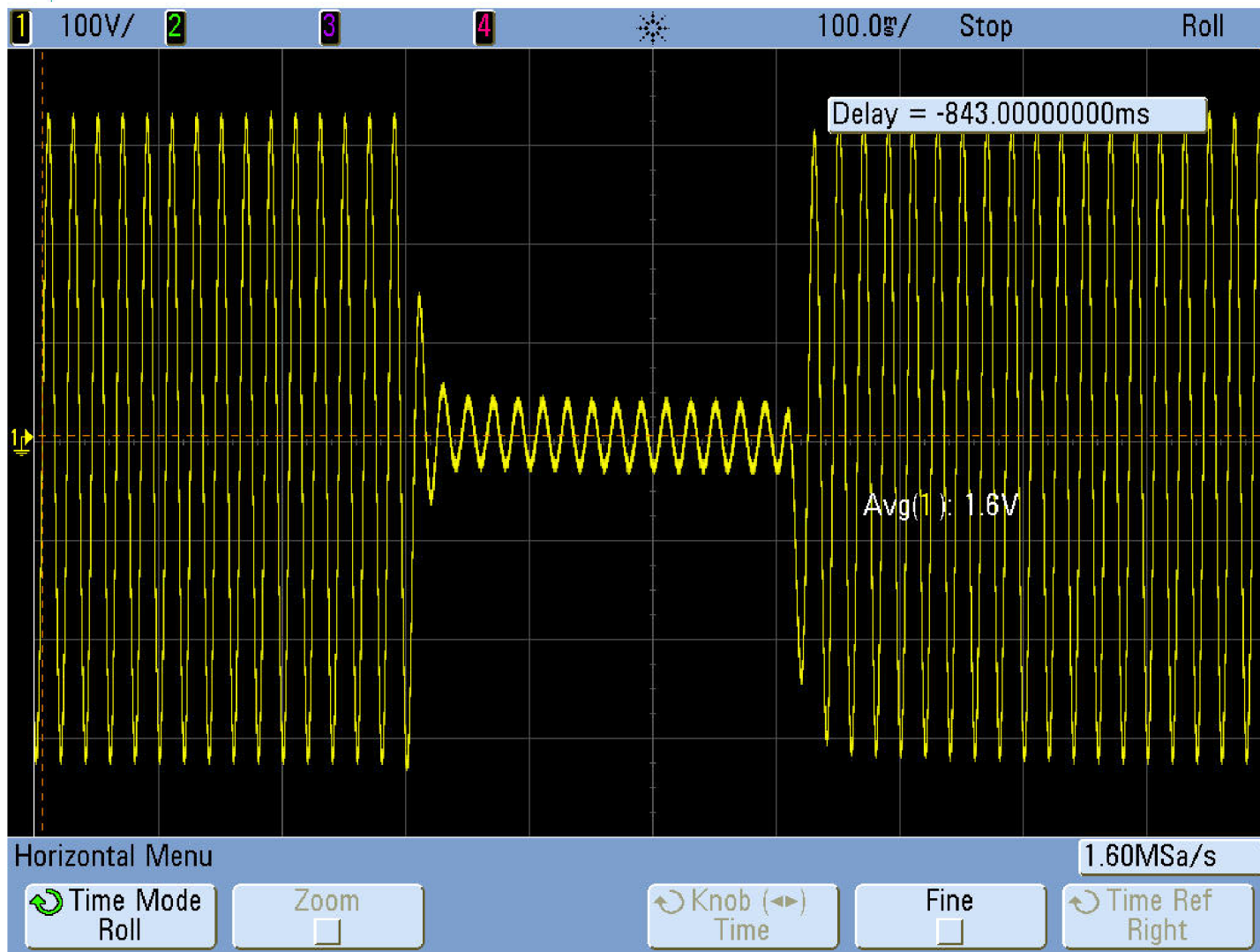
Obr. B.6: Zachycený pokles napětí osciloskopem Agilent.
