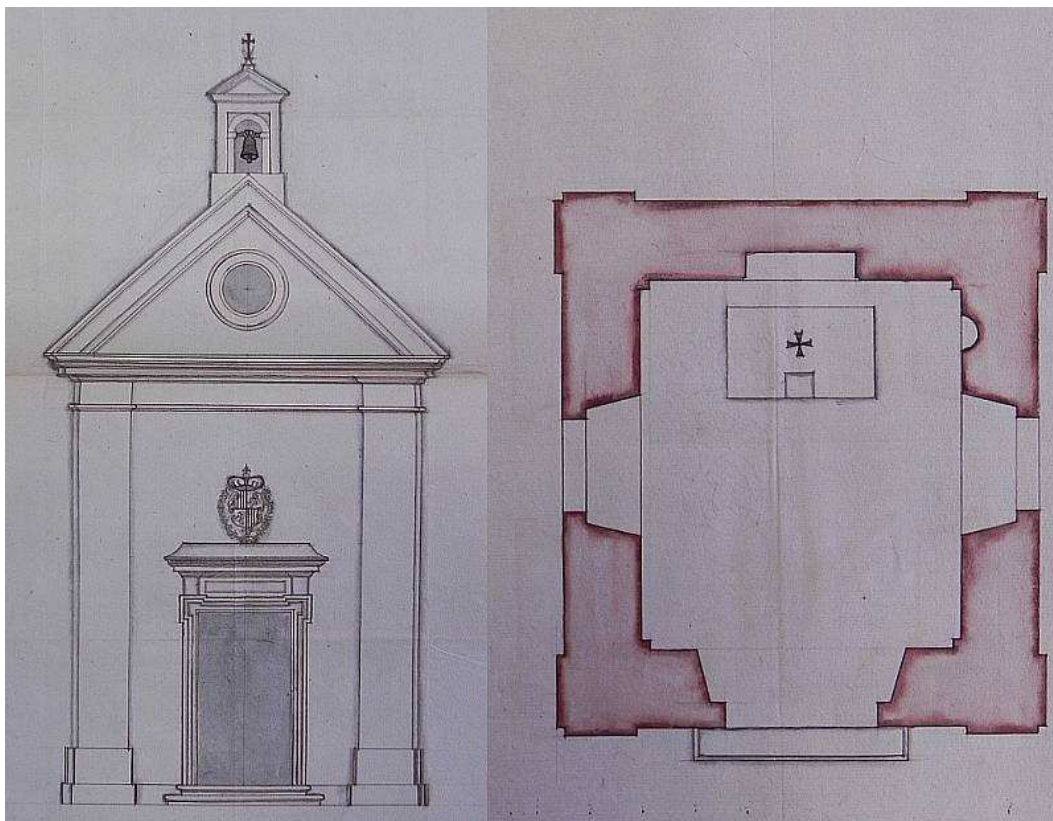
30. Giacomo Antonio de Maggi, nárys a půdorys kaple pro Libníč, 1691
