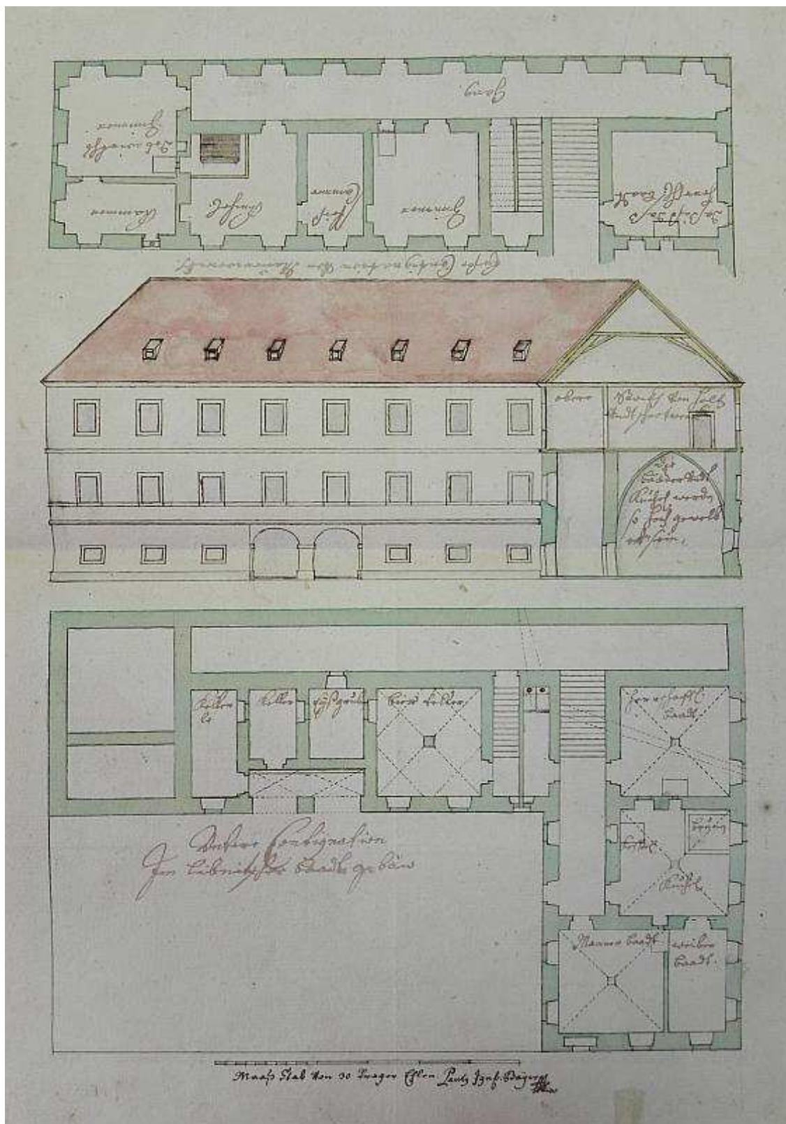
39. Pavel Ignác Bayer, plán lázní v Libníči – zdola sklep/přízemí, nárys nádvořího průčelí/řez křídlem s pramenem a koupelnami, půdorys zvýšeného přízemí, 1719
