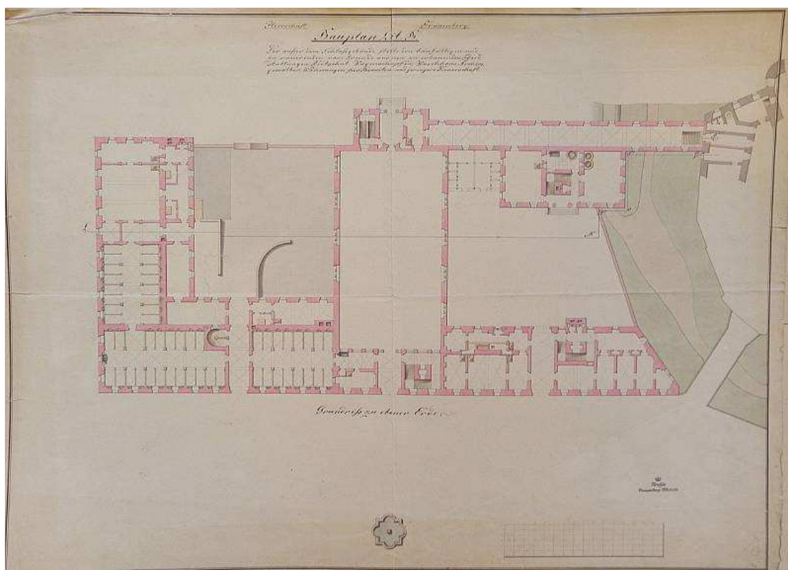
18. Vincenc Rohrbacher, Návrh nové budovy stáji a jízdní v předzámčí, před 1833
