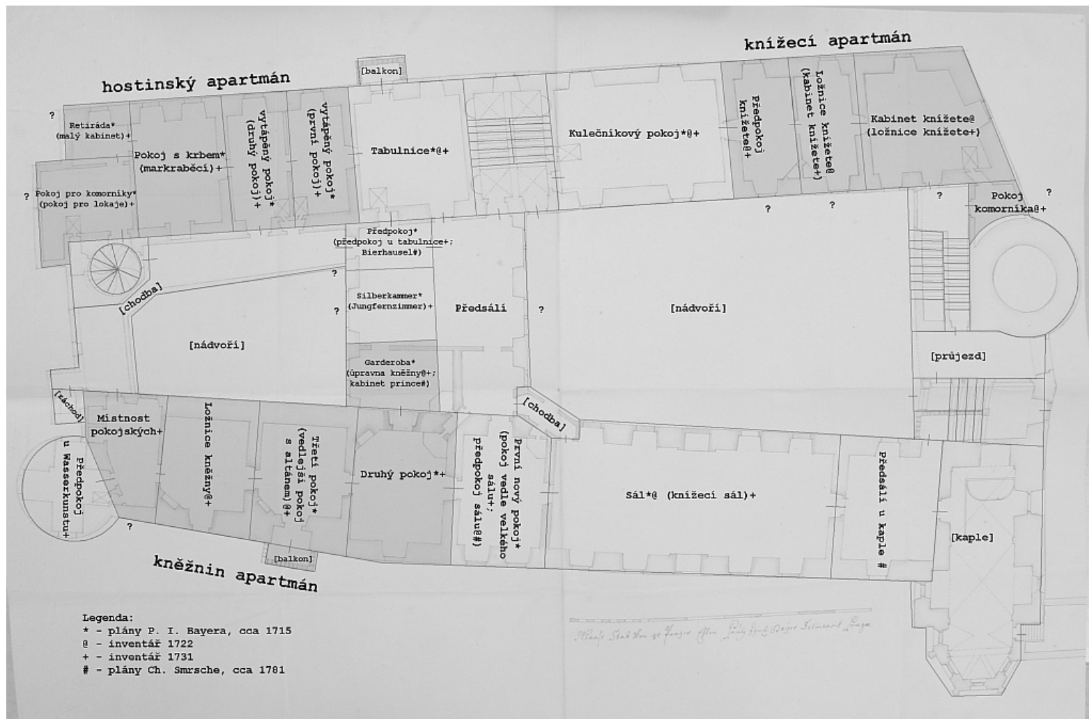
21. Hypotetická rekonstrukce členění piana nobile (otazníky – nejasné určení s možným odlišným členěním prostor; šedě zvýrazněny apartmány včetně pokojů služebných)
