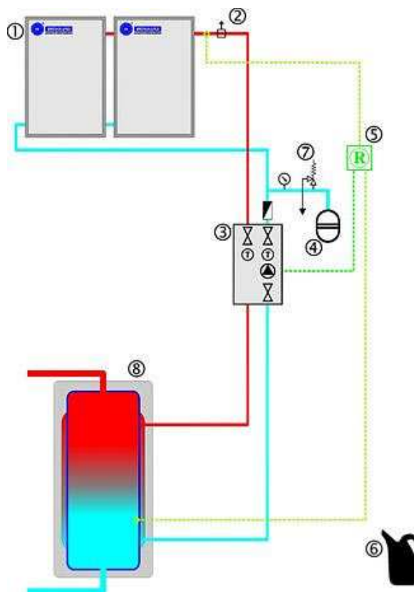
Obr.17: Hnaný solární systém [12]
