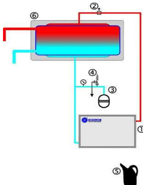
Obr.16: Samotížný solární systém [12]
