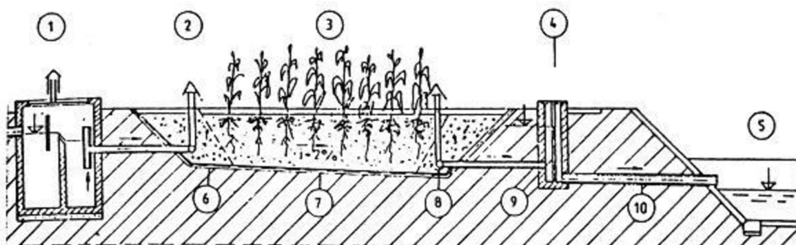
Obrázek 1: Možné uspořádání KČOV
