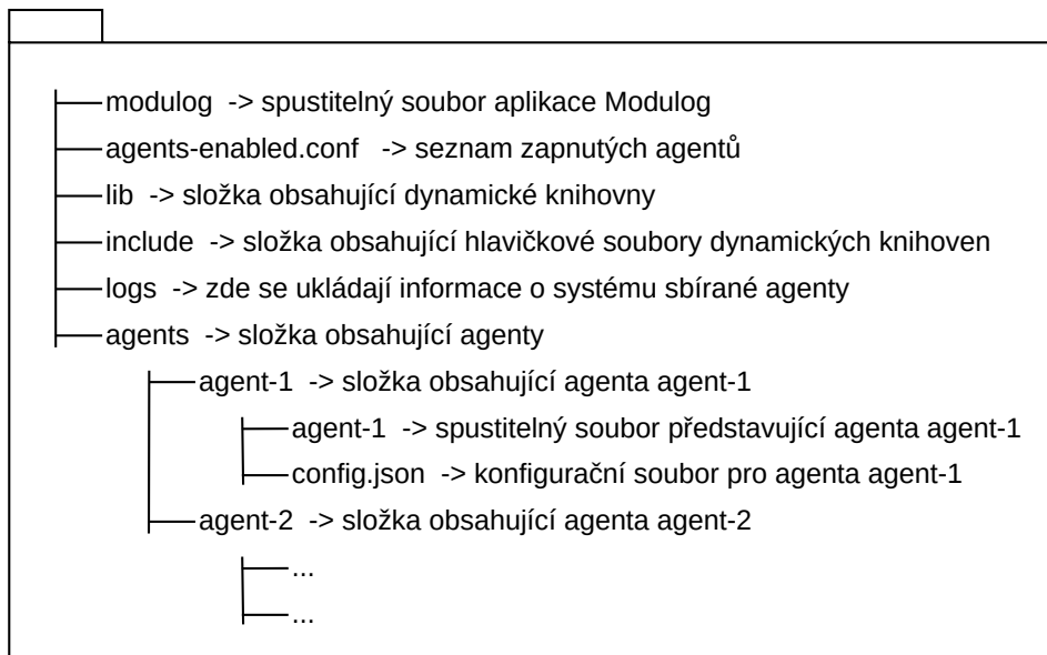
Obrázek 4.3: Struktura balíčku aplikace Modulog
