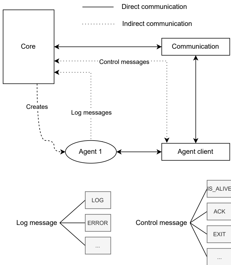
Obrázek 3.2: Architektura systému
