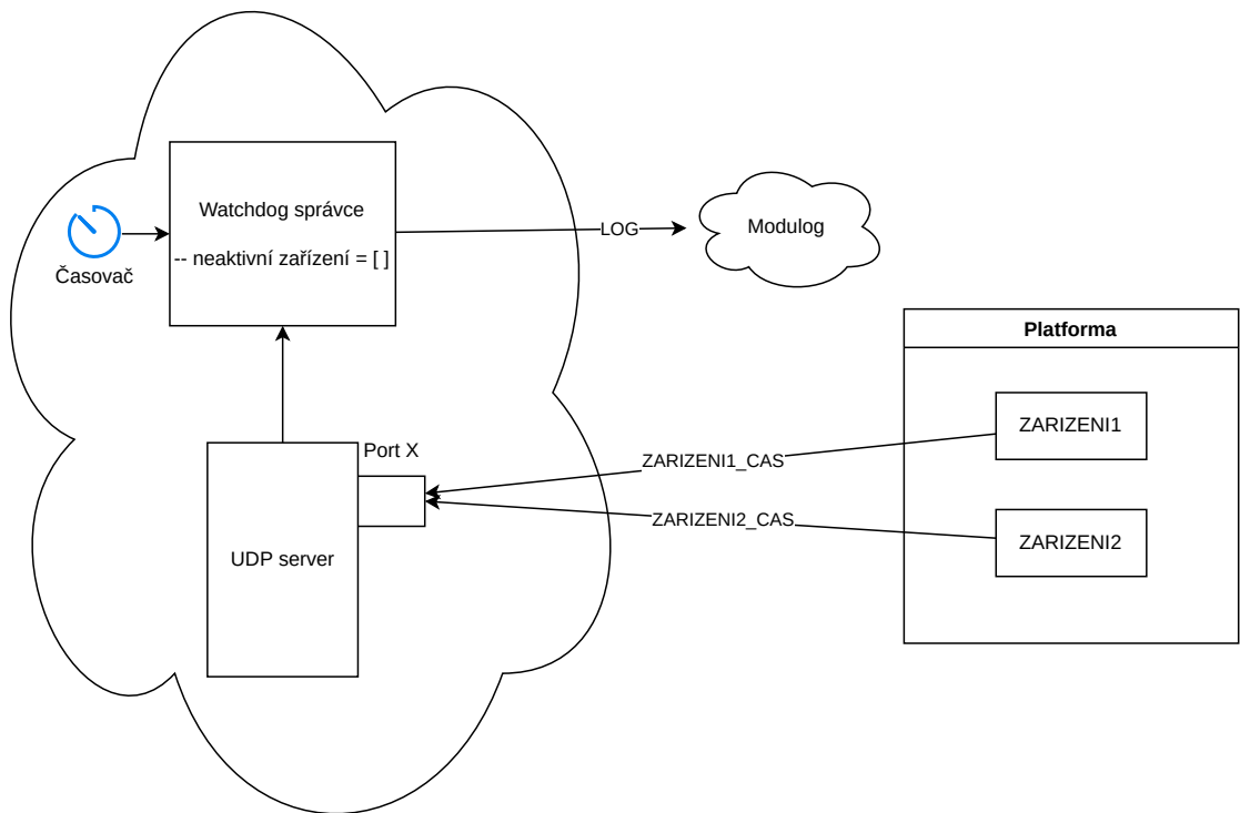
Obrázek 4.2: Zakomponování watchdog agenta do celého systému
