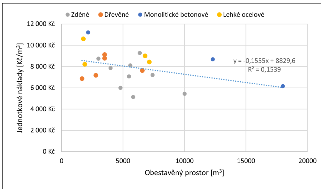
Obr. 18. Graf závislosti obestavěného prostoru a jednotkových nákladů [Kč/m 3 ]
