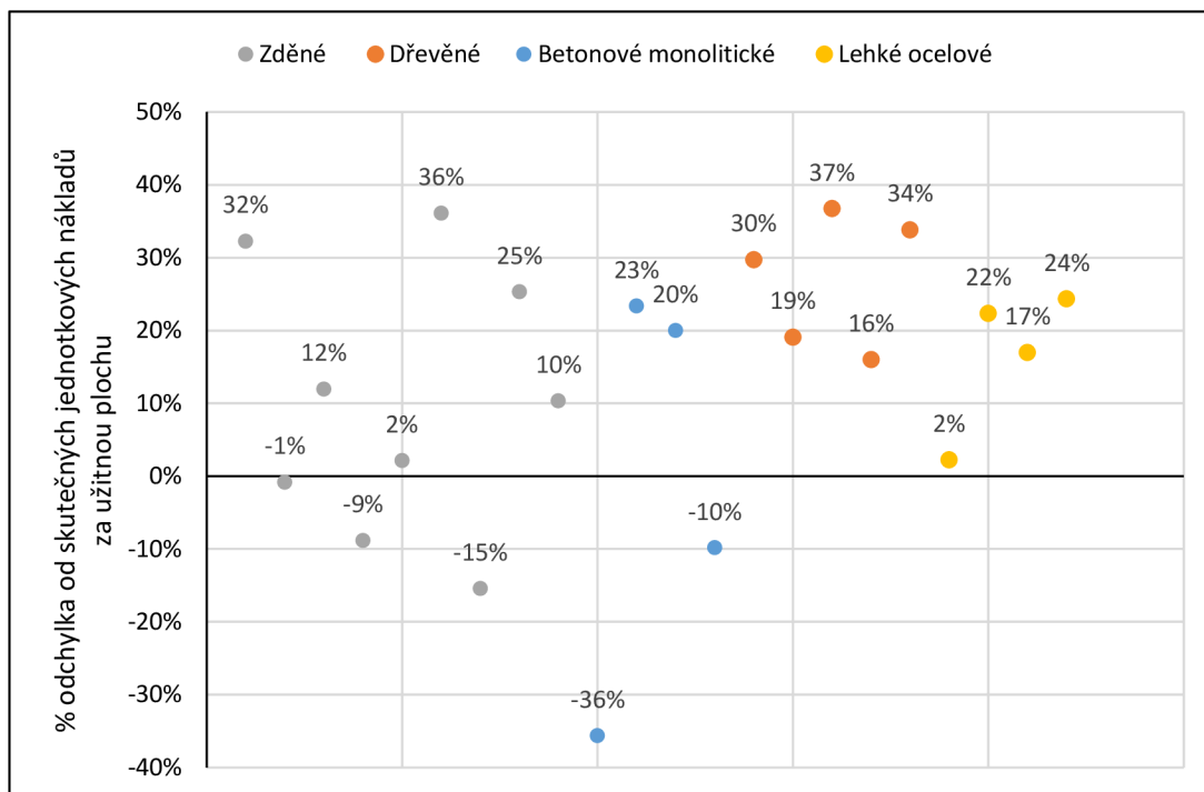
Obr. 21. Graf odchylek THU od skutečných jednotkových nákladů za užitou plochu u jednotlivých vzorků
