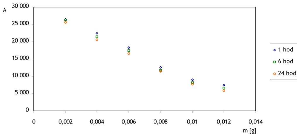
Obr. 5.4: Graf závislosti plochy píku pentachlorofenolu na množství použitého lignitu pro koncentraci PCP 5 \text{ mg}\cdot\text{l}^{-1}
