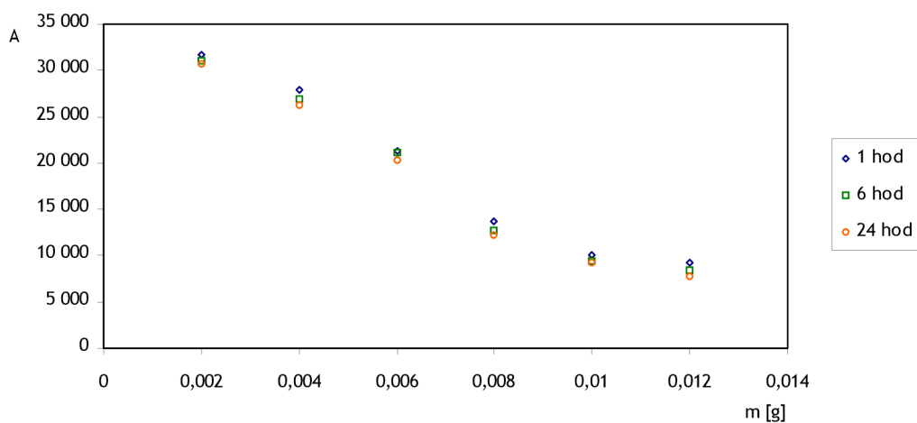
Obr. 5.5: Graf závislosti plochy píku pentachlorofenolu na množství použitého lignitu pro koncentraci PCP 6 \text{ mg}\cdot\text{l}^{-1}
