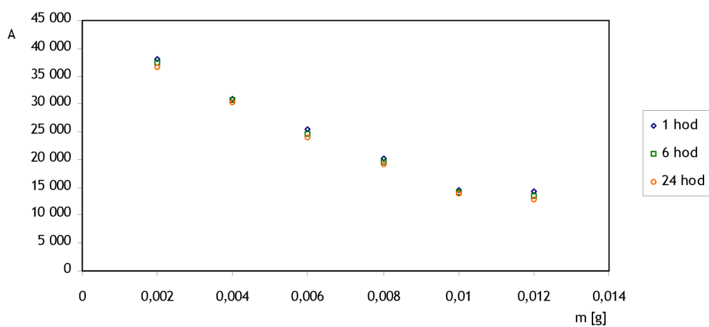
Obr. 5.7: Graf závislosti plochy píku pentachlorofenolu na množství použitého lignitu pro koncentraci PCP 8 mg·l -1
