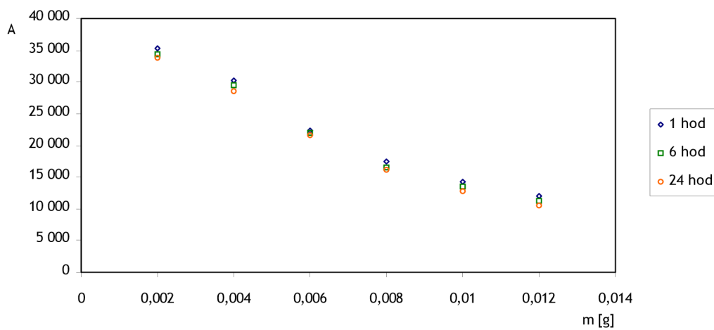
Obr. 5.6: Graf závislosti plochy píku pentachlorofenolu na množství použitého lignitu pro koncentraci PCP 7 mg·l -1
