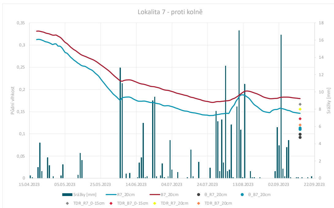
Obrázek 25: Porovnání naměřených vlhkostí mezi senzory TMS-4, objemových vlhkostí z odebraných válečků a naměřených vlhkostí pomocí metody TDR na lokalitě 7 v hloubkách 0 až 15 cm a 20 cm pod povrchem
