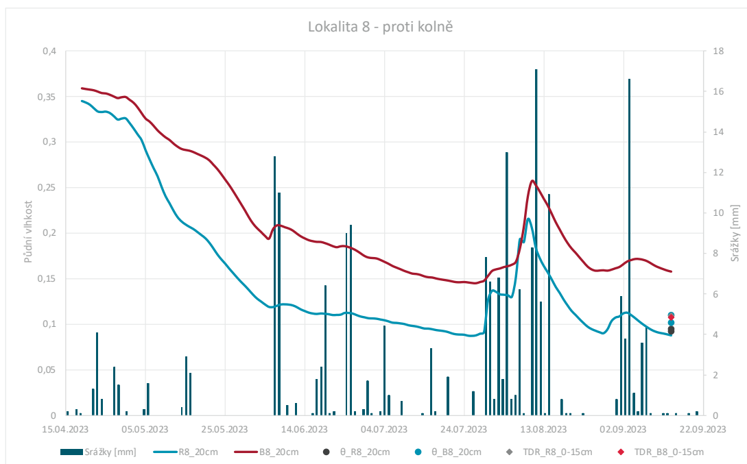
Obrázek 26: Porovnání naměřených vlhkostí mezi senzory TMS-4, objemových vlhkostí z odebraných válečků a naměřených vlhkostí pomocí metody TDR na lokalitě 8 v hloubce 20 cm pod povrchem
