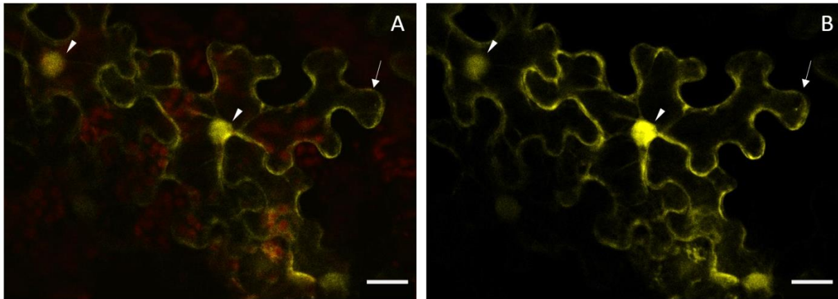
Obrázek 19: Fúzní protein YFP-MMK3 exprimovaný v epidermálních buňkách listů N. benthamiana transientně transformovaných bakterií A. tumefaciens nesoucí konstrukt AtUBQ10::YFP:cMMK3 použitý jako kontrola transformace. Snímky byly pořízeny konfokálním mikroskopem třetí den po transformaci, snímek A) spojení kanálů YFP+RFP+DAPI; B) kanál YFP použití Z-stack. Měřítko = 20 \mu\text{m} ; šipky označují specifický signál; trojúhelníky označují jádro.
