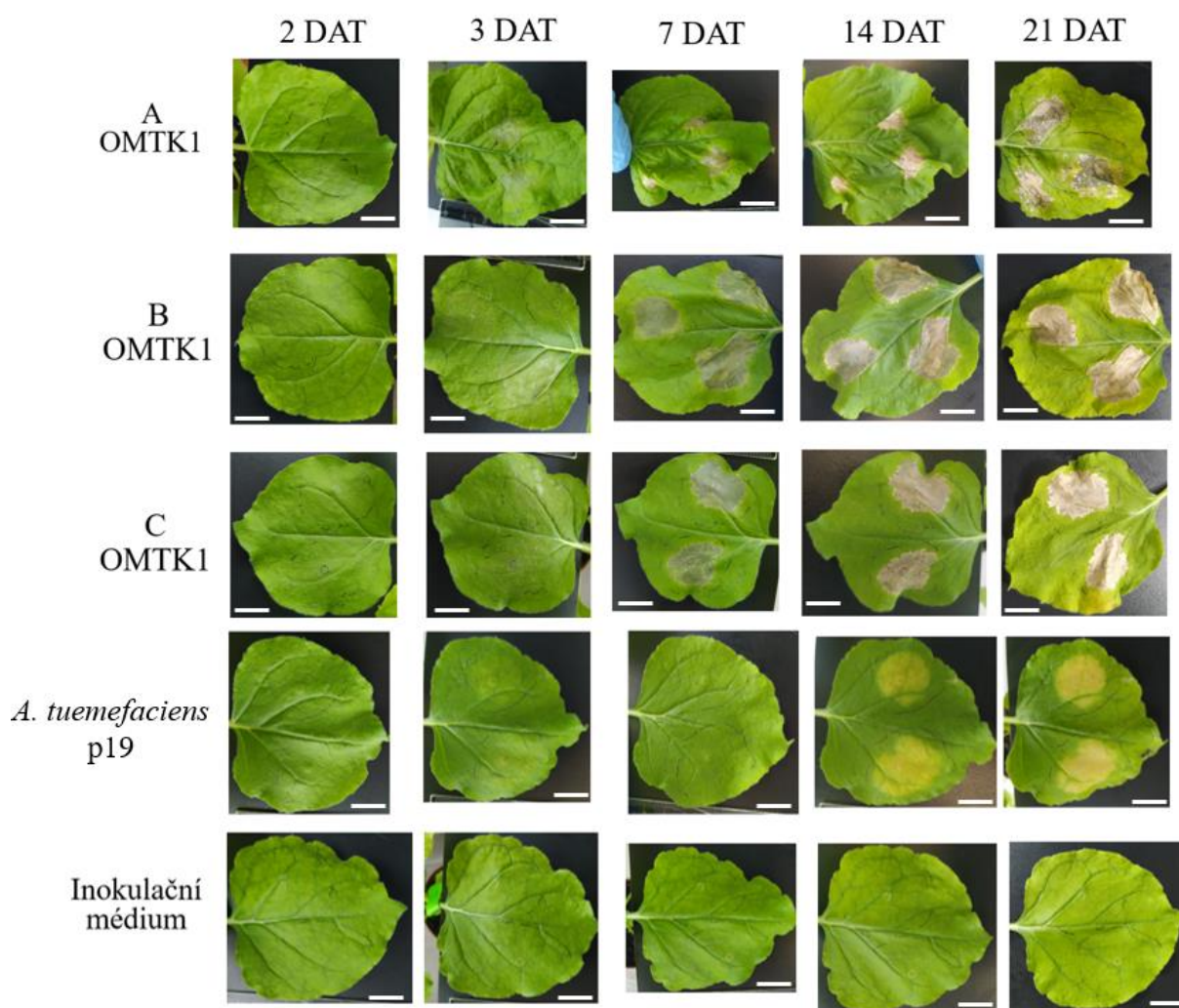
Obrázek 21: Fenotypová analýza listů N. benthamiana po transientní transformaci konstruktem AtUBQ10::YFP:cOMTK1 indukujícím zvýšenou expresi proteinu YFP-OMTK1. Jako kontrola byly použity buňky A. tumefaciens nesoucí konstrukt p19 a inokulační médium bez přidaných bakterií. Snímky byly pořízeny 2, 3, 7, 14 a 21 dní po transformaci (DAT). Měřítko 1 cm.
