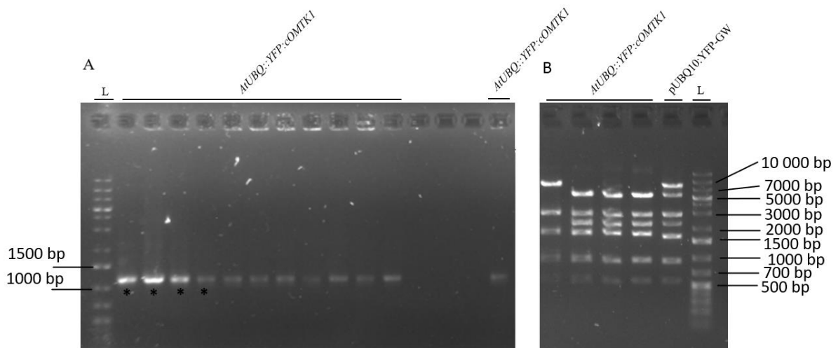
Obrázek 15: Selekcce kolonií E. Coli metodou PCR kolonií a restrikční štěpení plazmidu AtUBQ10::YFP:cOMTK1 . L- marker relativní molekulové hmotnosti. A) Selekcce kolonií E. Coli rekombinovaných tímto plazmidem; Hvězdičkou jsou označeny plazmidy, které byly použity pro následné restrikční štěpení; B) Restrikční štěpení rekombinovaného a prázdného plazmidu pomocí enzymu PstI.
