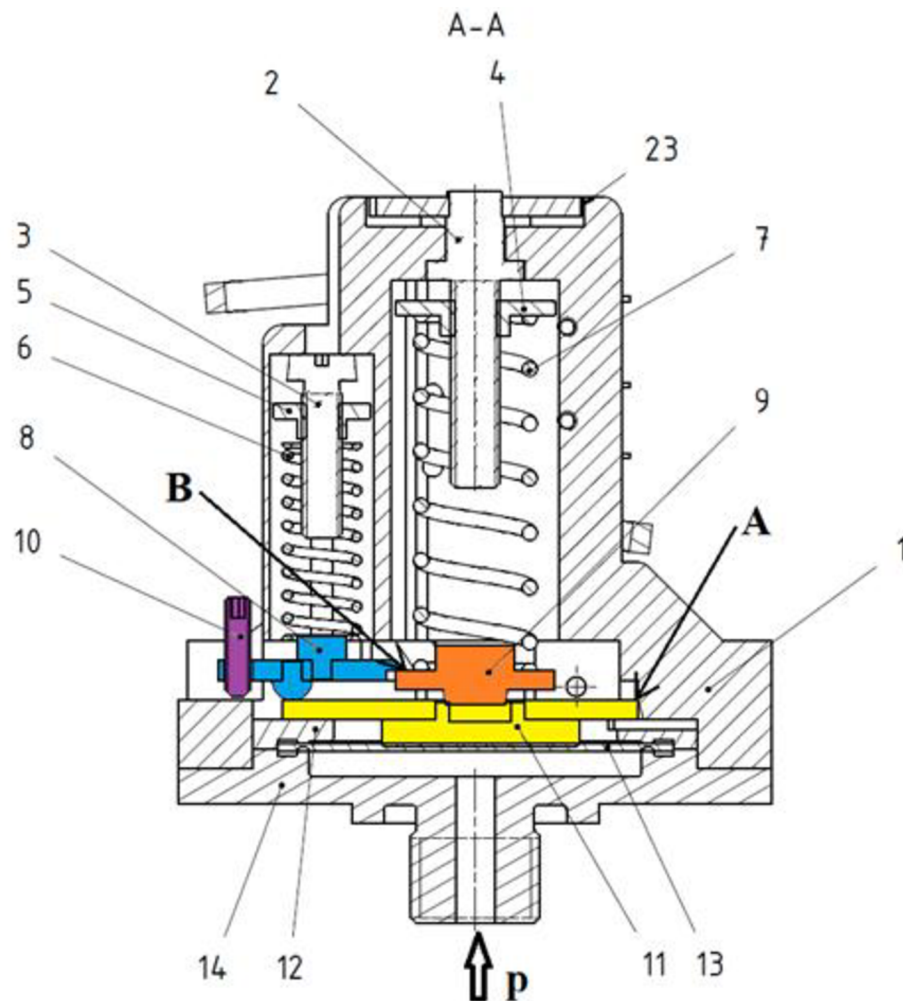
Obr. 25 – řez spínačem
