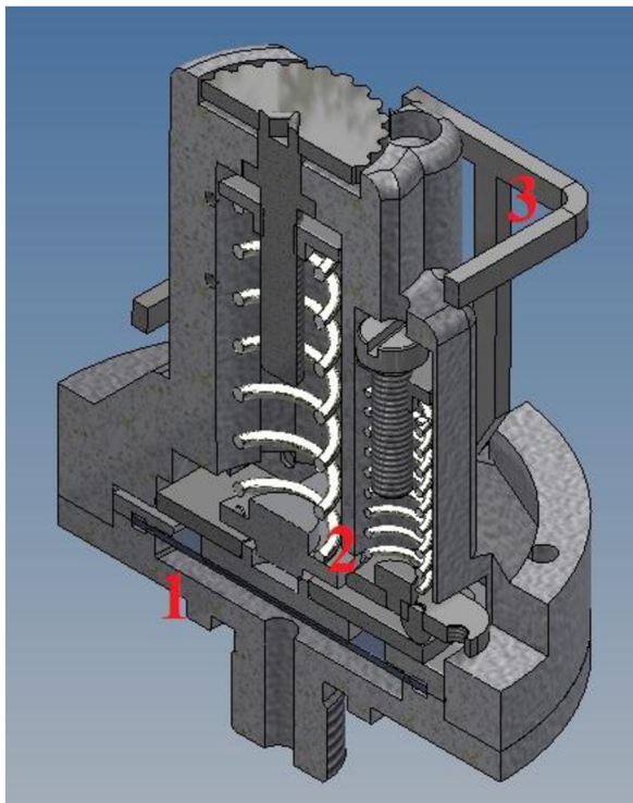
Obr. 14 řez spínačem
