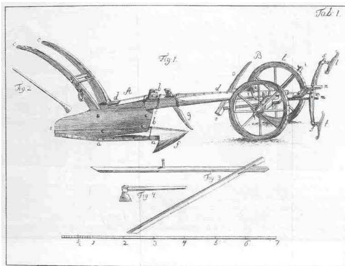
Oradlo z 18. století
