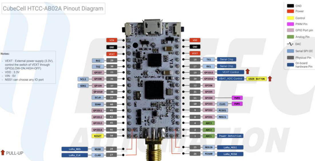
Obrázok 1.3 Pinout diagram použitej vývojovej dosky
