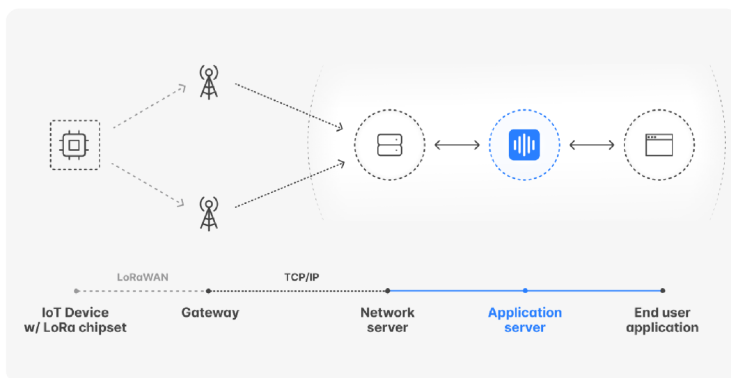
Obrázok 2.1 Schéma princípu fungovania siete LoRaWAN
