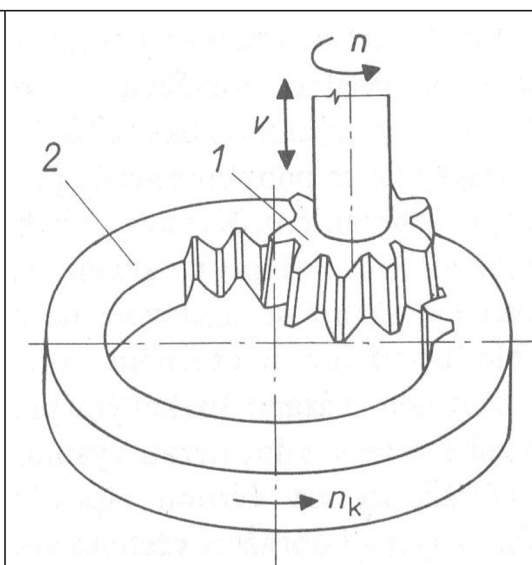
Obr. 1.13 Obrázení vnitřního ozubení kotoučovým nožem [2] 1 – kotoučový nůž, 2 – obrážené kolo
