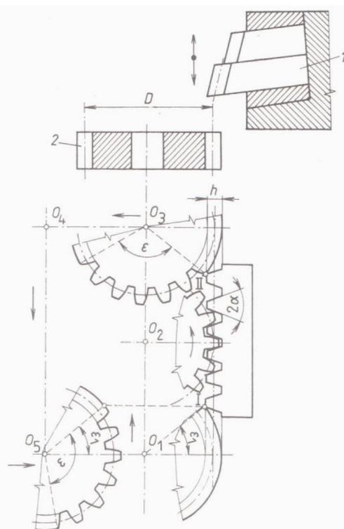
Obr. 1.10 Princip odvalovacího obrážení hřebenovým nožem [3] 1 – obrážecí hřeben, 2 – obrážené kolo
