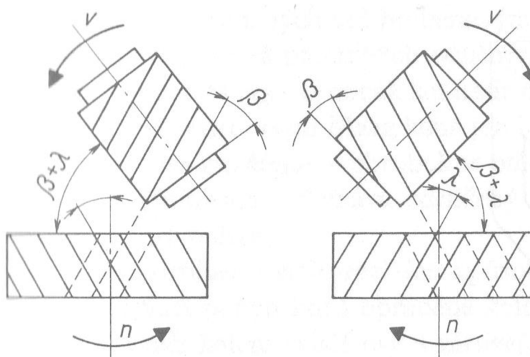
Obr. 1.10 Frézování šikmého ozubení s levým sklonem frézou pravochoudou a s pravým sklonem frézou levochoudou
