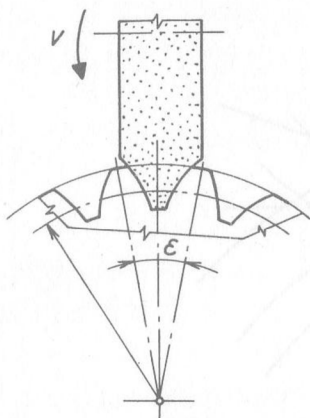
Obr. 1.18 Broušení zubů tvarovým kotoučem [2]
