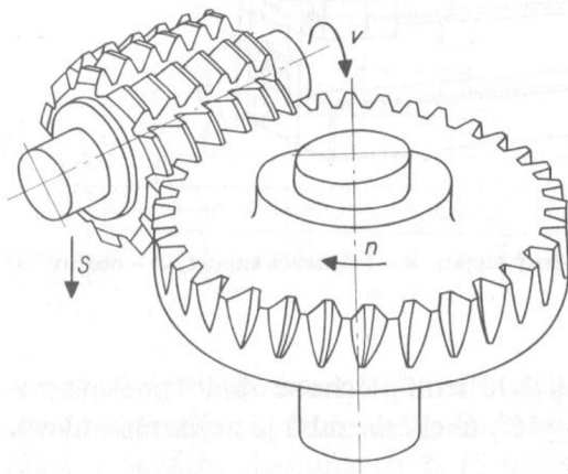
Obr. 1.4 Frézování přímých zubů [2]
