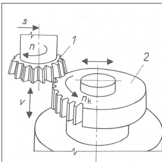
Obr. 1.12 Obrázení vnějšího ozubení kotoučovým nožem [2] 1 – kotoučový nůž, 2 obrážené kolo
