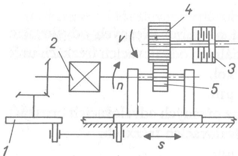
Obr. 1.23 Lapování ozubených kol [2]
