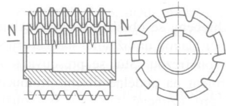
Obr. 1.5 Odvalovací fréza [3]
