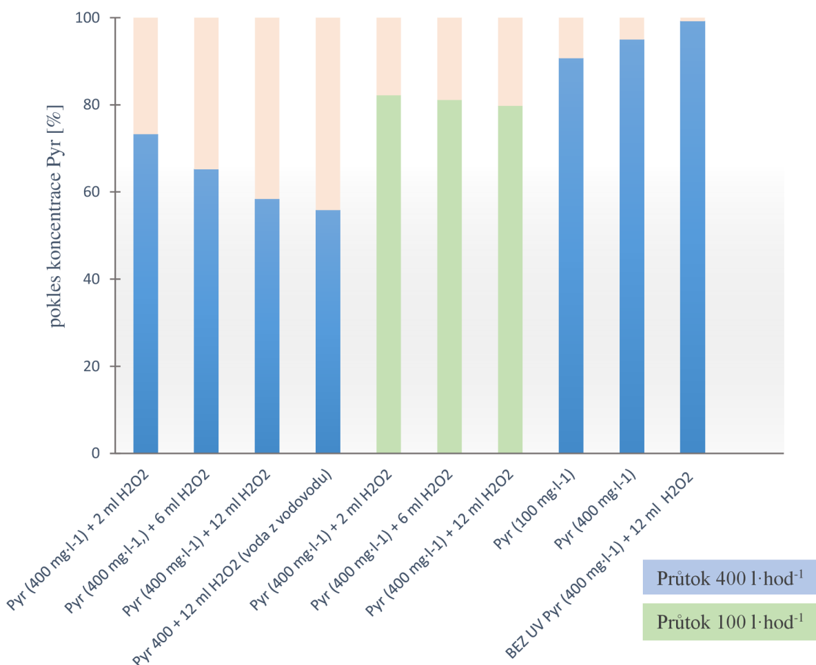
Graf 14: Porovnání účinnosti jednotlivých podmínek měření
