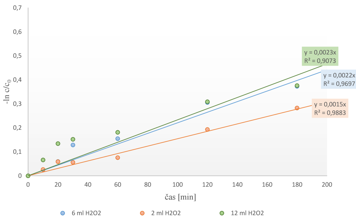
Graf 15: Porovnání rychlosti degradace pyridinu o počáteční koncentraci 400 \text{ mg} \cdot \text{l}^{-1} (5 l) s dávkou 2, 6 a 12 ml H_2O_2
