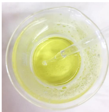
Obrázek 21: Zabarvení roztoku po 180 minutách experimentu
