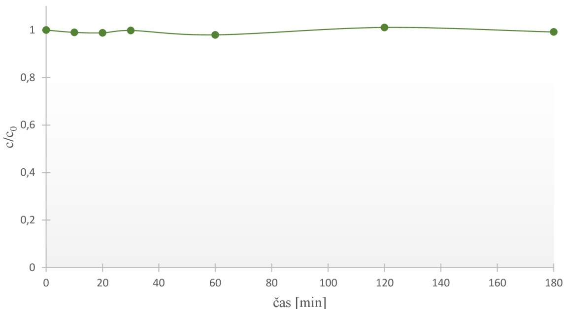
Graf 13: Časový průběh poklesu koncentrace pyridinu při dávce H_2O_2 12 ml, průtok 400\ l\cdot hod^{-1} , bez použití UV záření
