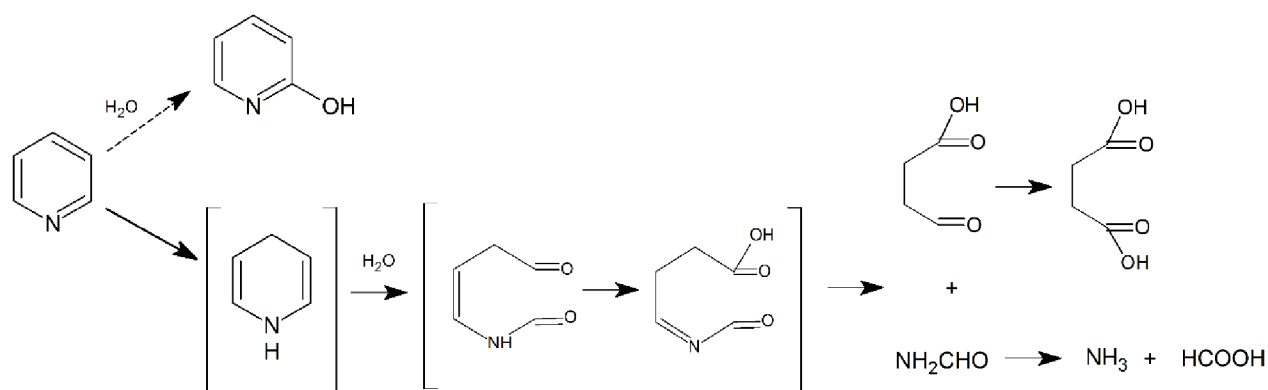
Obrázek 11: Degradace pyridinu působením UV záření o vlnové délce \lambda = 254 nm, převzato a upraveno dle [58]
