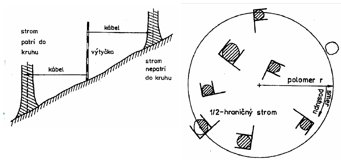
Vytyčení kruhové zkusné plochy
