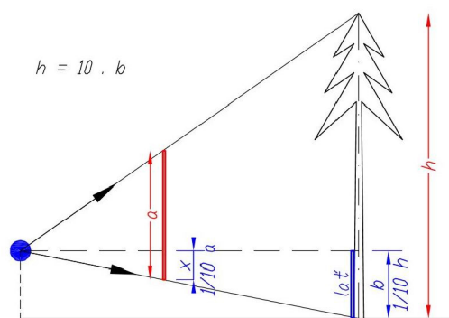
Princip měření výšek - geometrický (Christenův) varianta Christenova výškoměru
