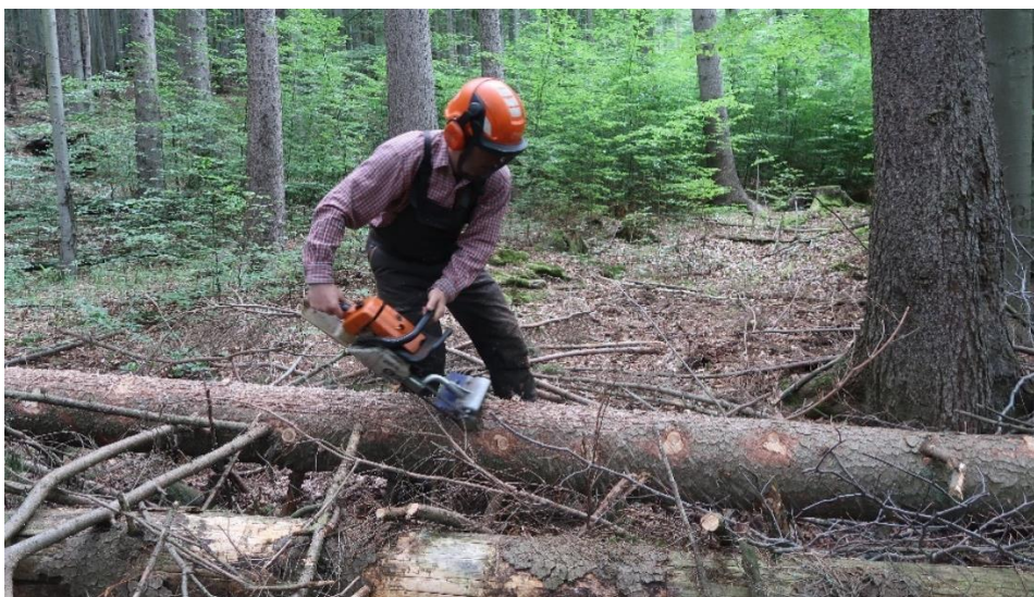
Obrázek 5: Provádění drážkové asanace pomocí motorové pily s nástavcem (foto: M. Havira)
