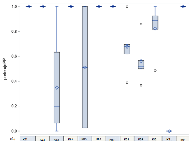
Graf 2: Podíl stání s pravou hrudní končetinou hlouběji pod tělem z celkového času rozkročených stání („preferujePP“; doplněk do 1,0 tvoří podíl stání s levou hrudní končetinou hlouběji pod tělem)
