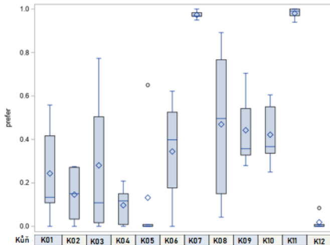
Graf 1: Podíl rozkročených postojů z celkové doby stání („prefer“) u 5 měření každého z koní (N = 12)
