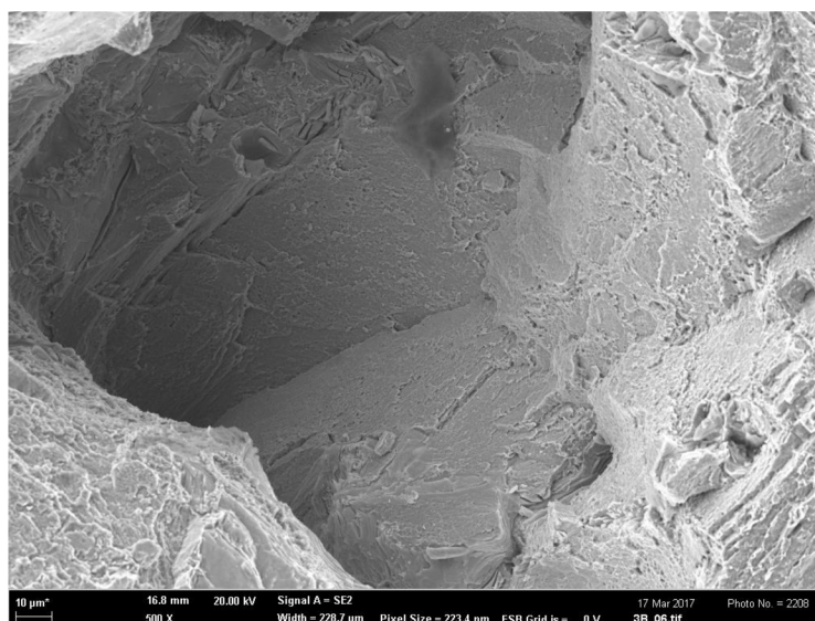
Obr. 58: Lomová plocha vzorku po tahové zkoušce, vz. blok po TZ
