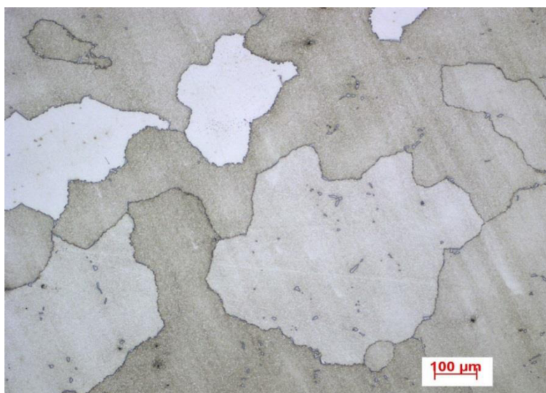
Obr. 32: Karbidy vyloučené po hranicích zrn, s disperzí fáze \gamma' , vz. blok HIP+TZ
