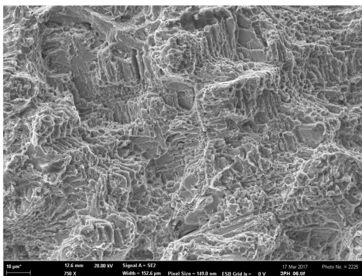
Obr. 43: Lomová plocha vzorku po tahové zkoušce, vz. předlitý HIP+TZ
