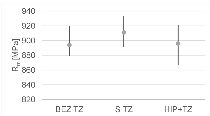
Graf 8: Srovnání pevnosti v tahu vzorků „komolokužel“
