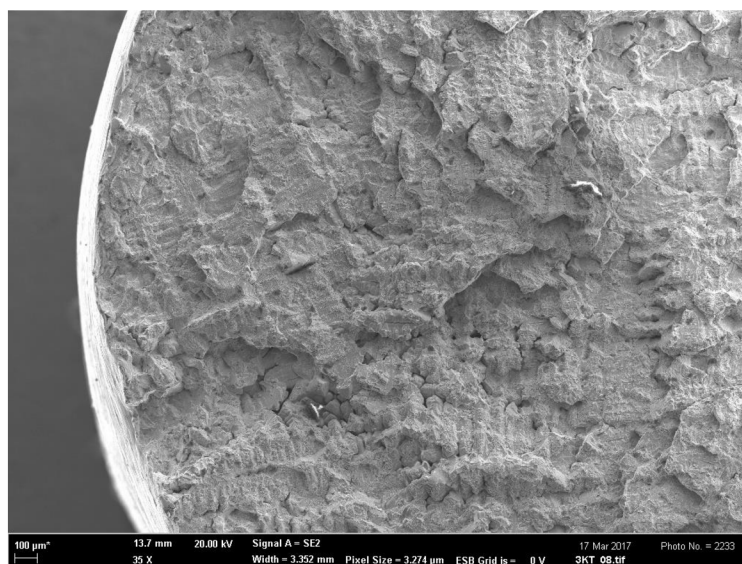
Obr. 47: Lomová plocha vzorku po tahové zkoušce, vz. komolokužel po TZ
