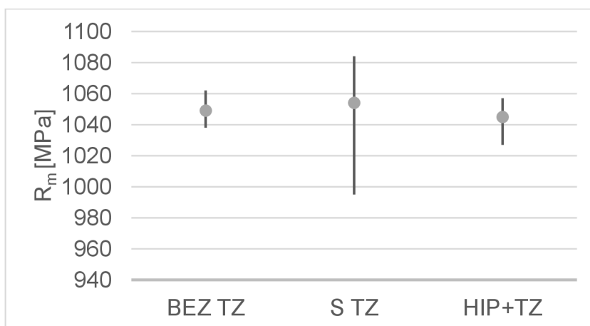
Graf 7: Srovnání pevnosti v tahu vzorků „předlitý“
