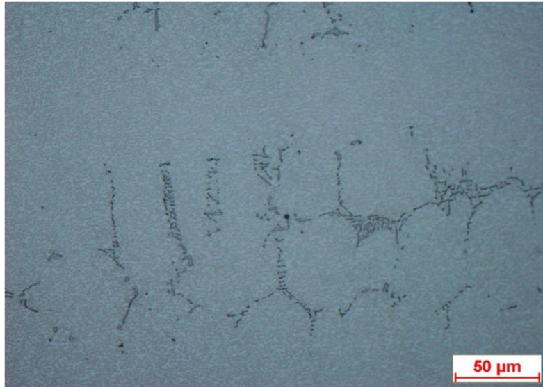
Obr. 21: Karbidy typu MC v mezidendritických prostorech, vz. předlitý HIP+TZ
