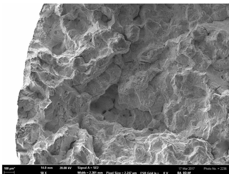
Obr. 53: Lomová plocha vzorku po tahové zkoušce, vz. blok bez TZ
