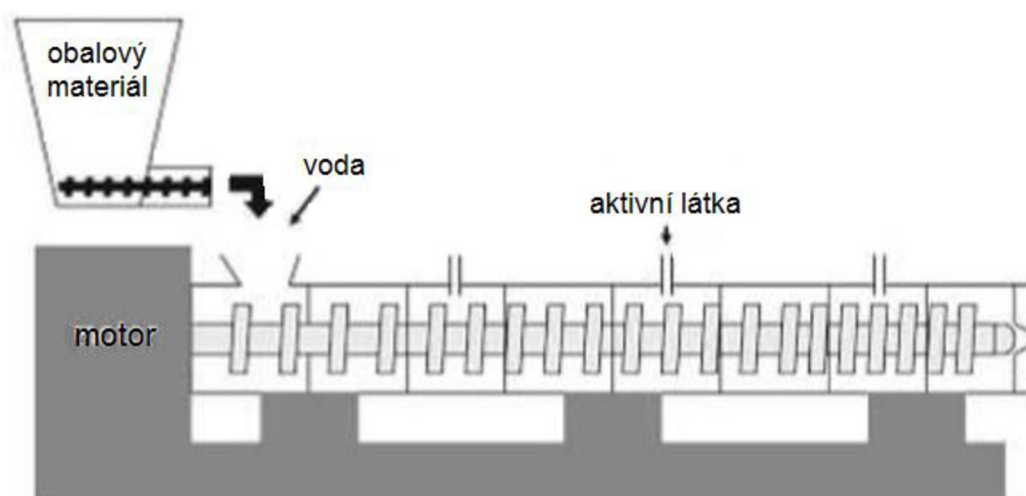
Obrázek 6: Extrudér [31]
