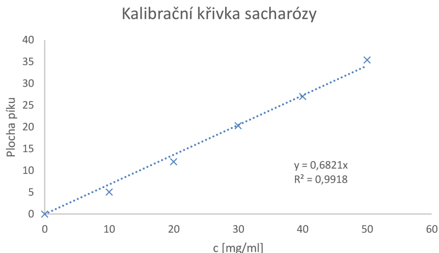
Graf 5: Kalibrační křivka sacharózy stanovená na NH 2 koloně
