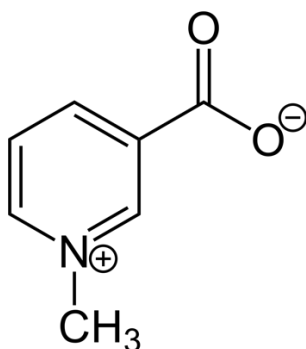
Obrázek 3 Strukturní vzorec trigonellinu ( https://cs.wikipedia.org )
