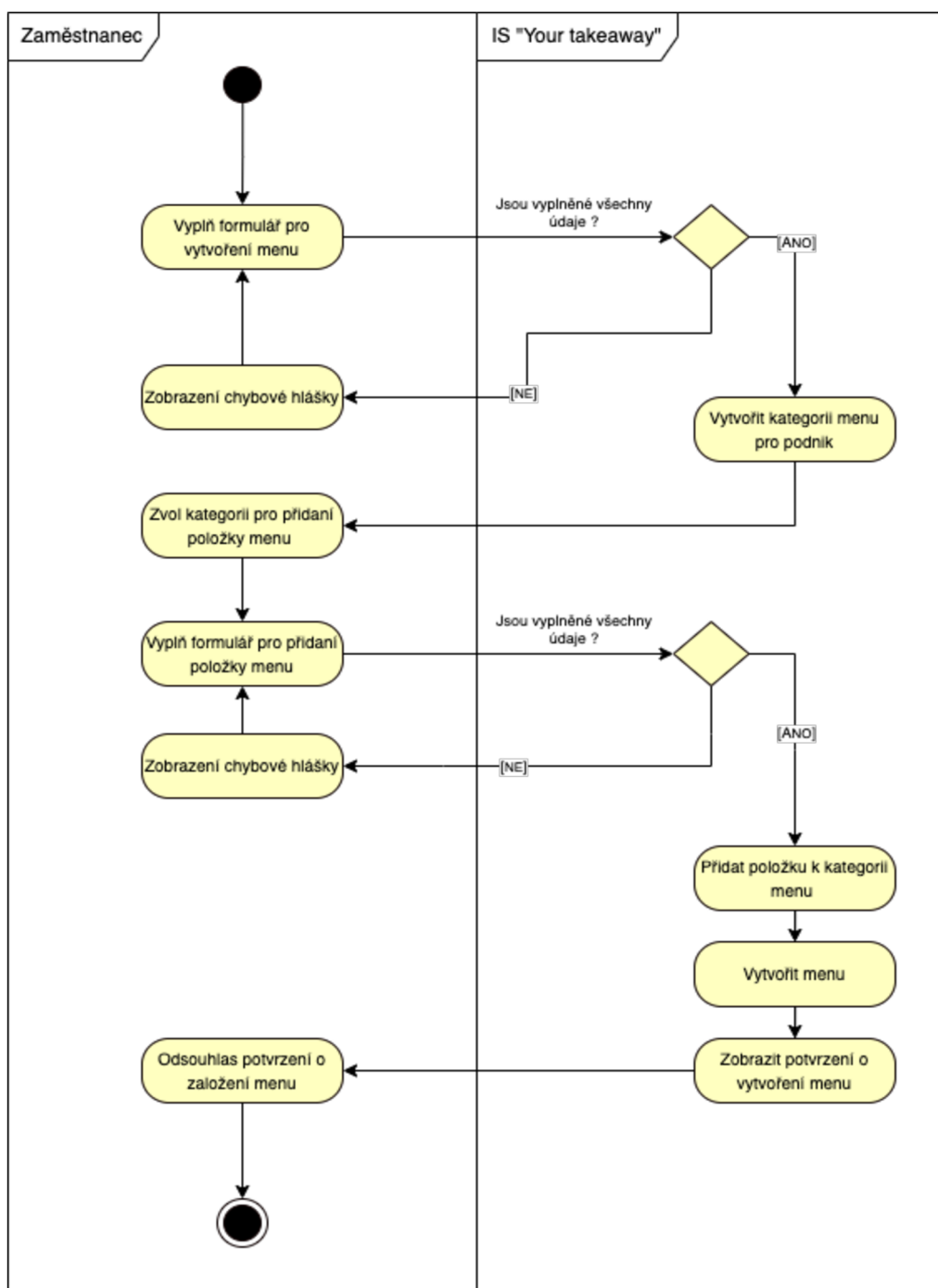
Obrázek 25: Aktivita diagram: Přidání menu (Zdroj: Vlastní tvorba)
