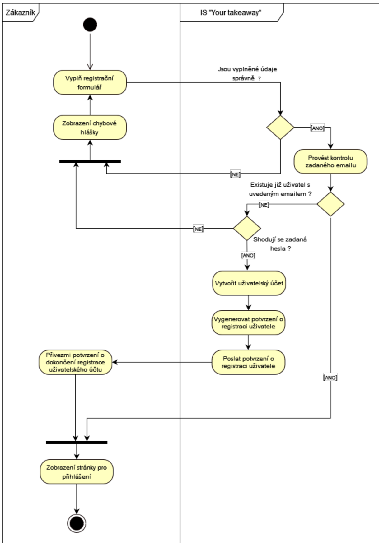
Obrázek 28: Aktivitní diagram: Registrace zákazníka (Zdroj: Vlastní tvorba)
