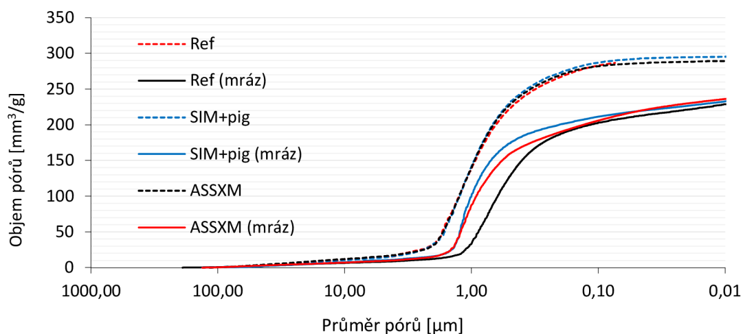
Graf 6 Distribuce pórů střepe nehydrofobizovaného a hydrofobizovaného střepe
