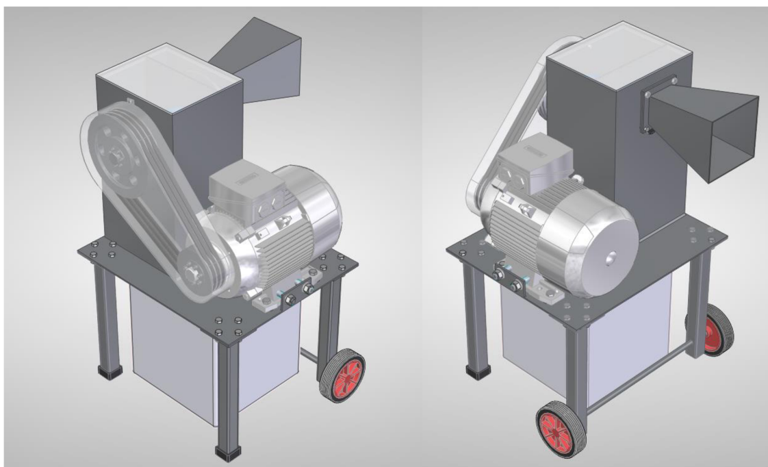
Obr. 48 3D model zahradního drtiče
