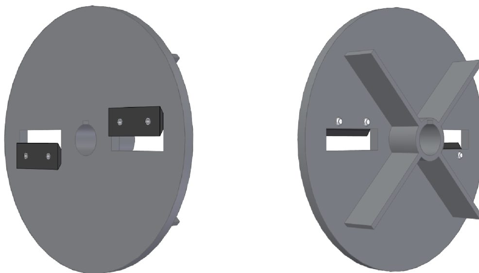
Obr. 47 Diskový sekací mechanismus
