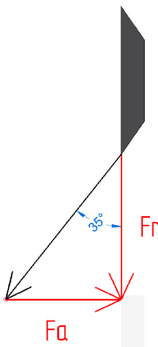
Obr. 37 Rozložení sil na noži sekacího mechanismu
