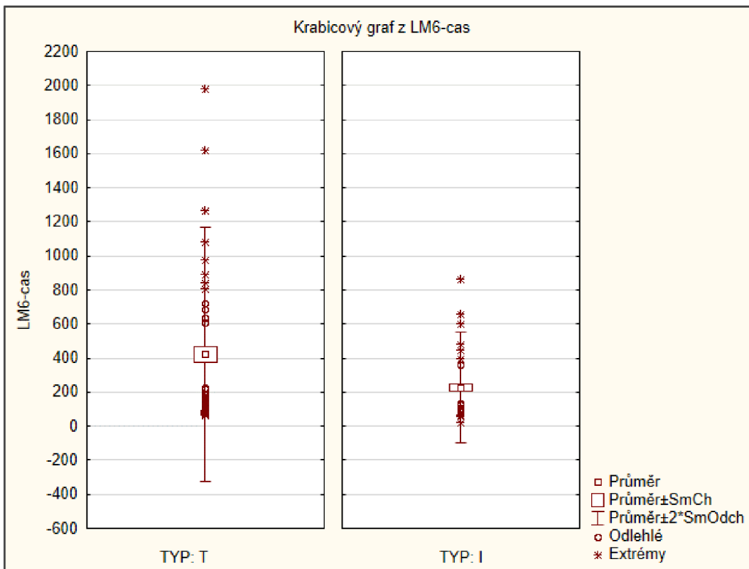
Graf 6 – Krabicový graf z LM6, hledisko čas, střední hodnota průměr
