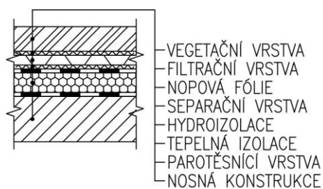
Obrázek 5-2: Schéma skladby STR-VEG
