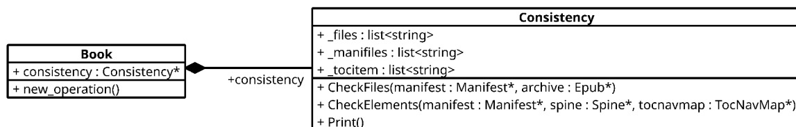
Obrázek 3.5: Diagram třídy Consistency .
