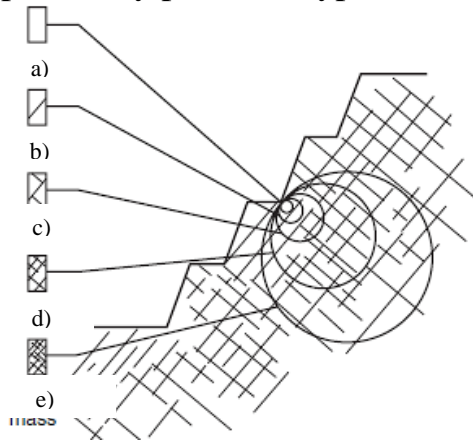
Obr.4 Idealizované schéma velikosti vzorku a přechodu od horniny a) celistvé; b) s jedním systémem puklin; c) se dvěma systémy puklin; s mnohočetným systémem puklin až ke e) zcela porušenému masivu (upraveno podle Wyllie 2014)
