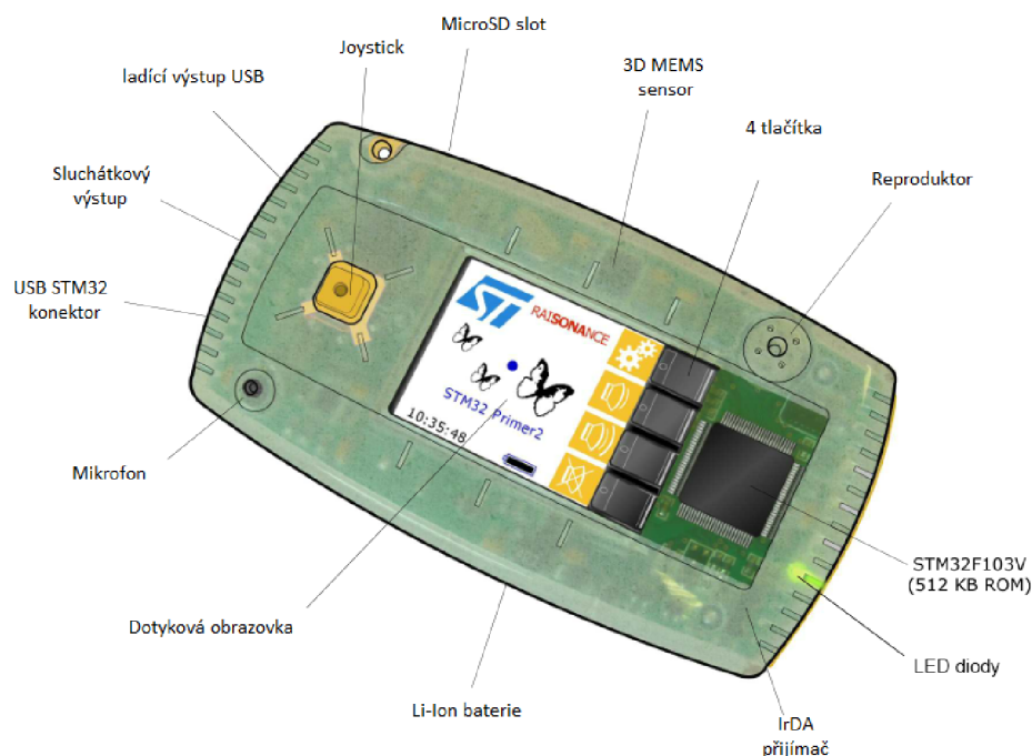
Obr. 2.7: Popis vývojového kitu STM32-Primer2
