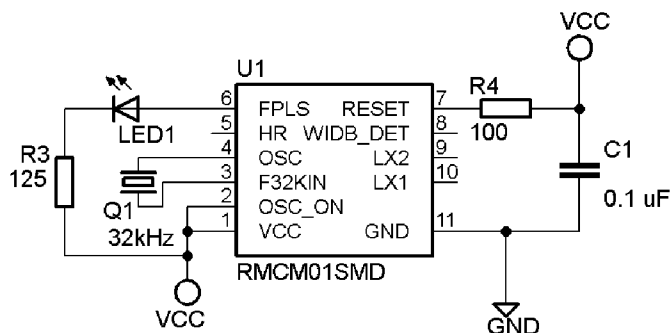
Obr. 3.2: Testovací schéma
