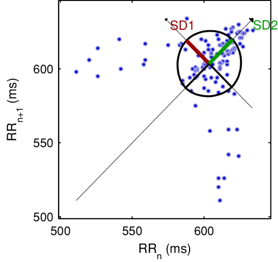
Obr. 2.4: Příklad Poincarého mapy
