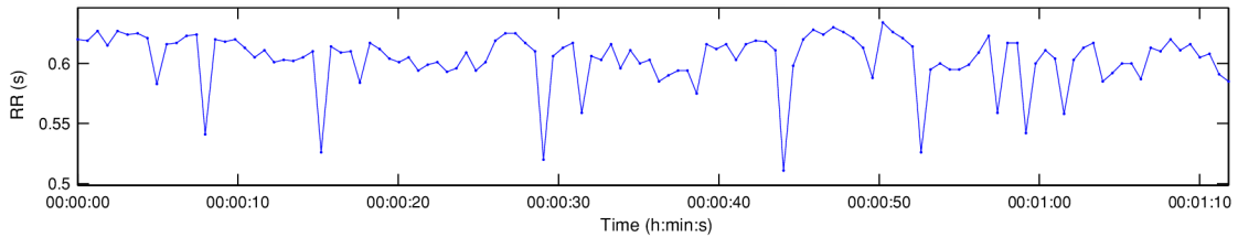
Obr. 2.3: Časový záznam délky RR intervalů
