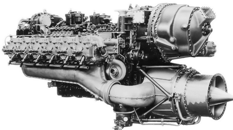
Obr. 2.14: Boční pohled na motor Napier Nomad II
