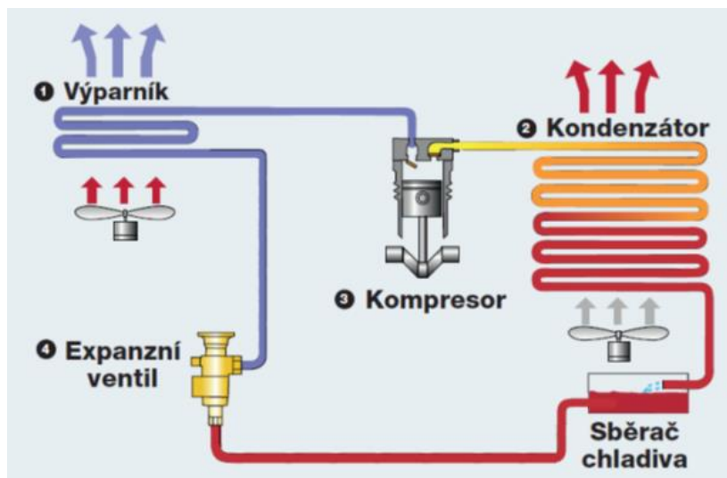
Obr. 3 - Schéma tepelného čerpadla [6]
