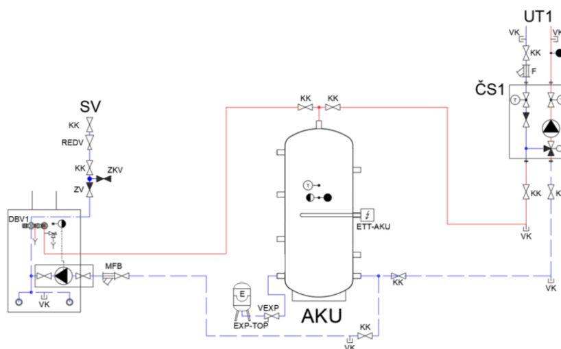
Obr. 7 - Schéma zapojení kotle a akumulární nádoby [Vytvořeno autorem]
