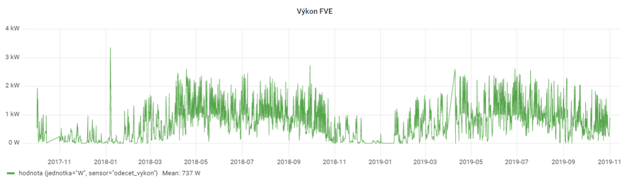
Graf 1 - Výkon FVE 2017-2019 [Vytvořeno autorem]
