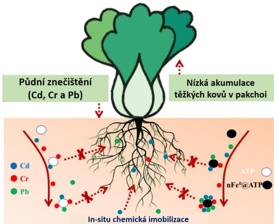
Obrázek 9 Schéma in-situ imobilizace Cd, Cr a Pb pomocí ATP a ATP@nZVI a jejich vlivu na akumulaci kovových kontaminantů zeleninou pakchoi upraveno dle Xu a kol. (2019).
