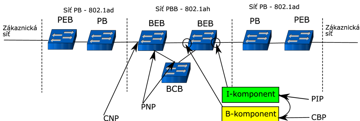
Obrázek 2.5: Zobrazení topologie PBBN s PBN
