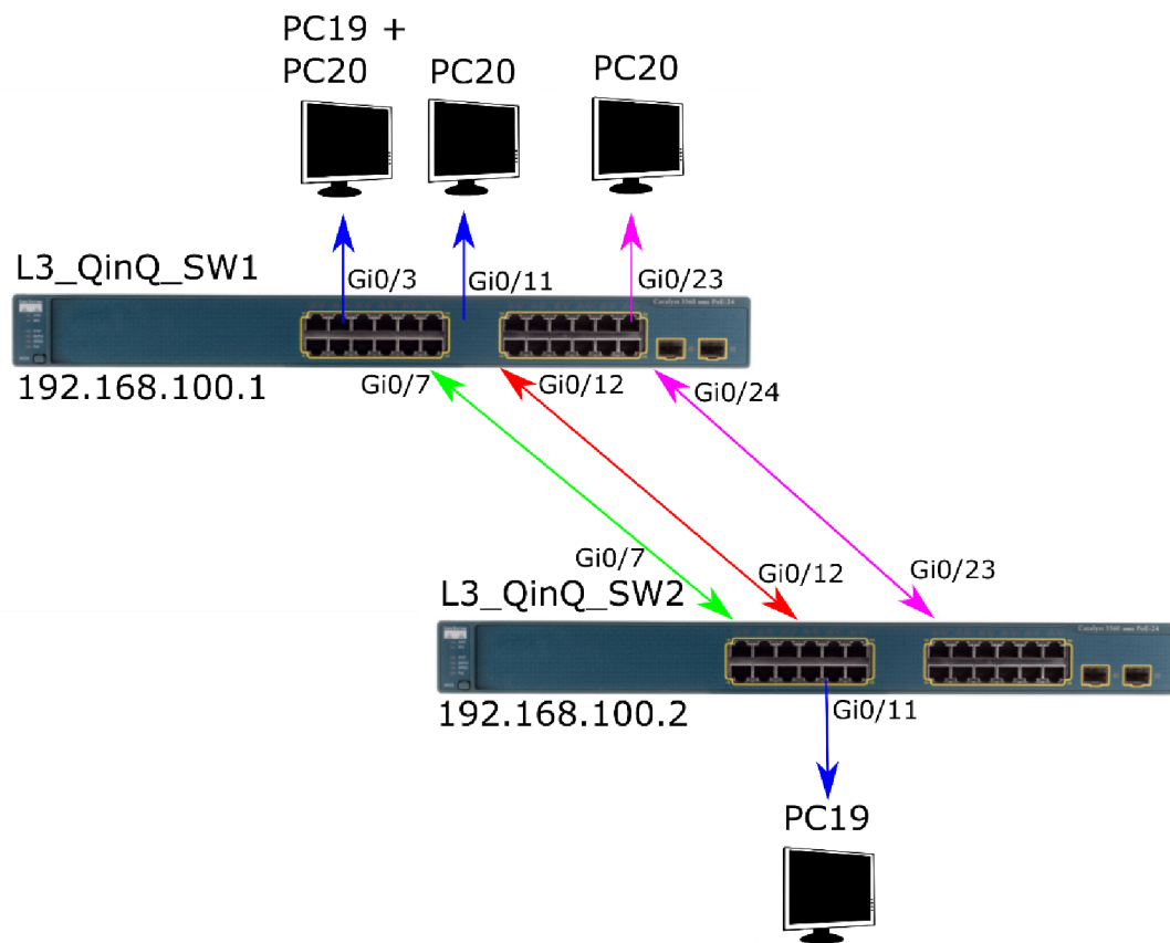
Obrázek 3.1: Zapojení laboratorní úlohy v učebně
