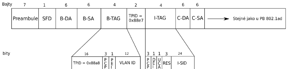
Obrázek 2.3: Formát Rámce PBB
