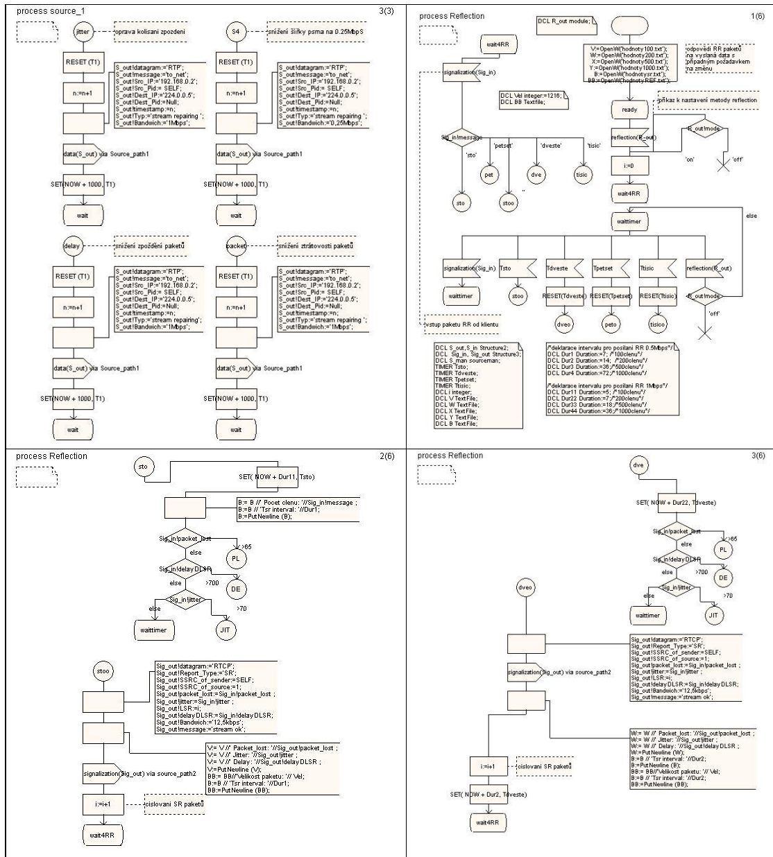
Obr. 33: Struktura procesu source_1 a ukázka struktury procedury Reflection
