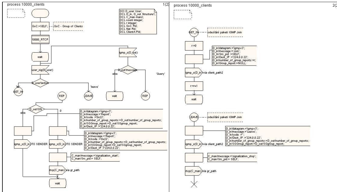
Obr. 28: Ukázka procesu řešení komunikací protokolu IGMPv3 v bloku clients
