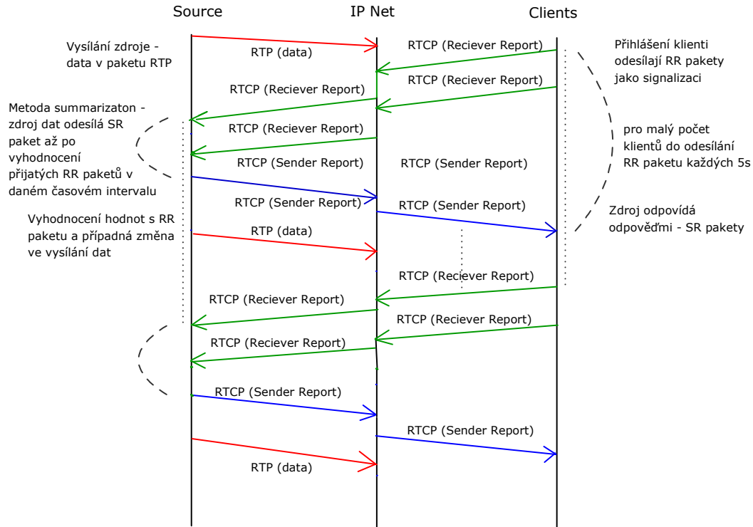
Obr. 19: Zasílání RR a SR paketů - metoda reflection
