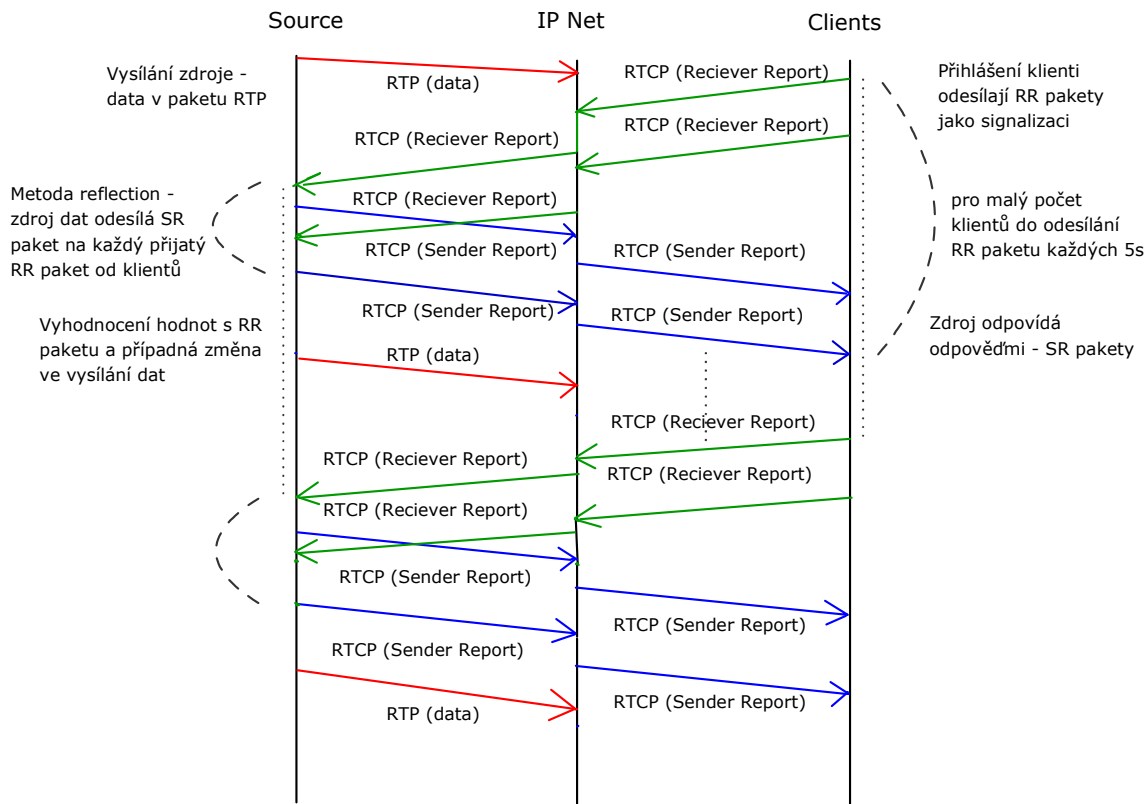
Obr. 18: Zasílání RR a SR paketů - metoda reflection
