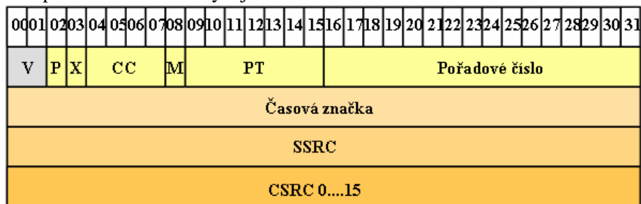
Obr. 10: Struktura protokolu RTP [4]
