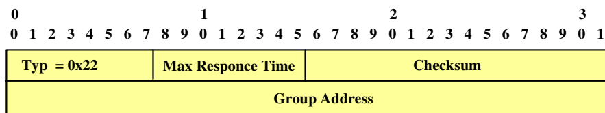
Obr. 6: Struktura zprávy IGMPv2 [12]
