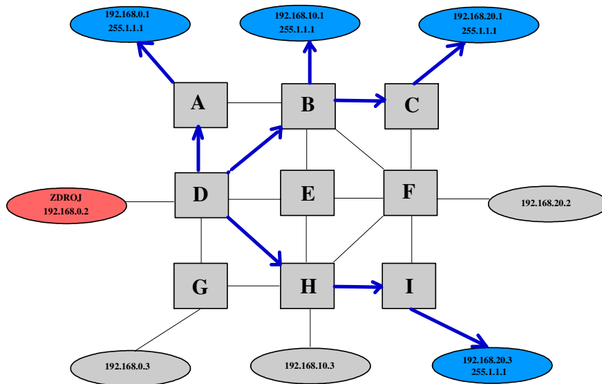
Obr. 2: Zdrojový strom [7]
