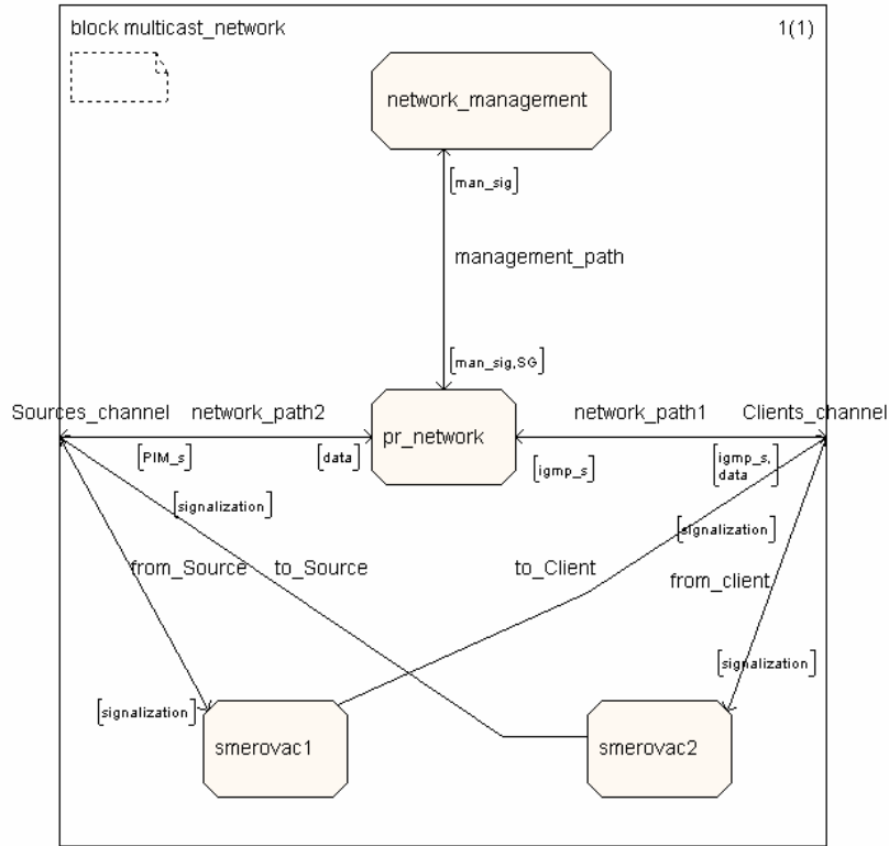
Obr. 30: Procesy tvořící blok multicast_network
