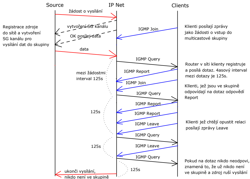
Obr. 17: IGMP zprávy
