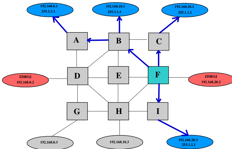
Obr. 3: Sdílený strom [7]
