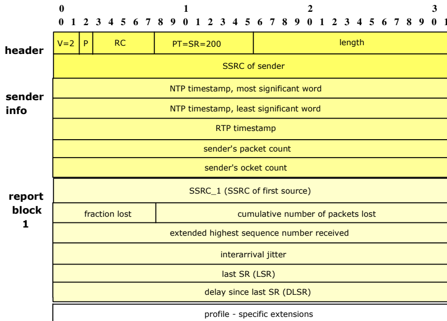
Obr. 12: Struktura paketu SR [16]
