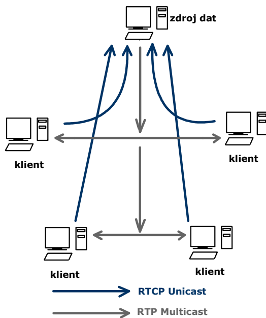
Obr. 14: Protokol RTP/RTCP v modelu multicastové komunikace SSM s unicastovým signalizačním kanálem [13]
