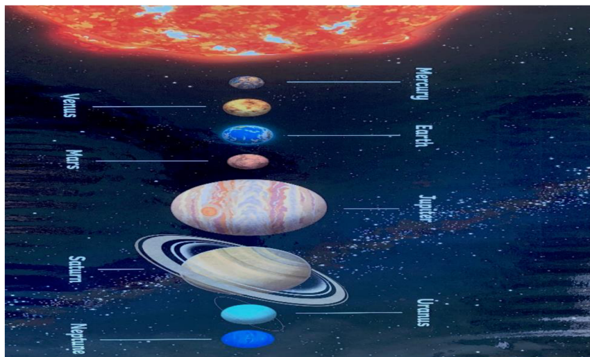
Obrázek 34: Sluneční soustava
