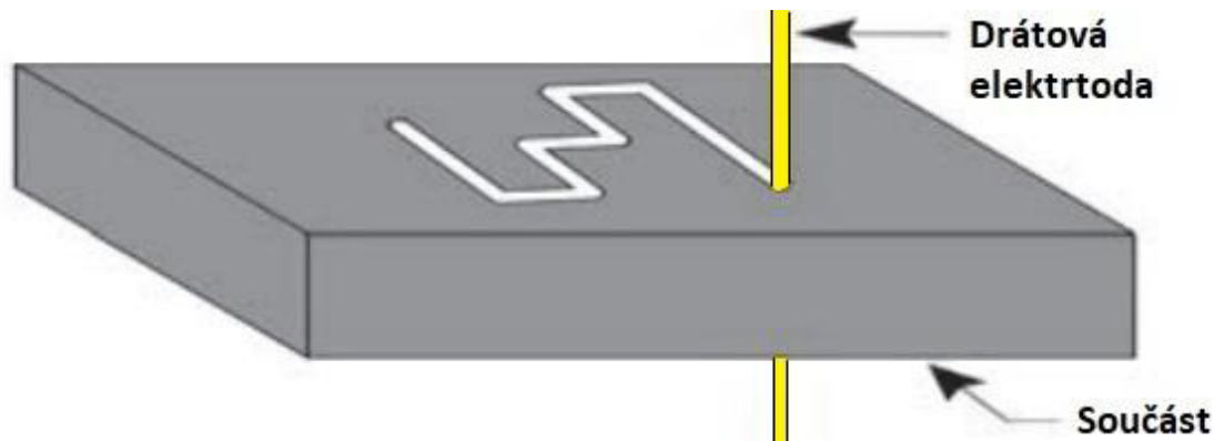
Obr. 3.1 Drátová metoda [21].
