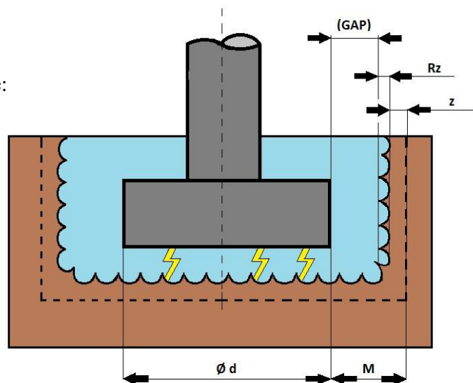
Obr. 2.22 Rozměr elektrody [7].
