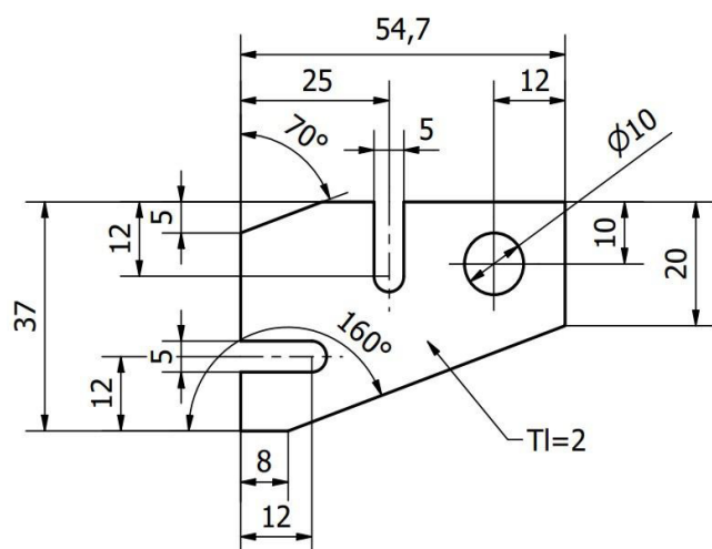
Obr. 4.3 Výkres výstřížku.
