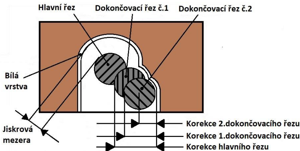
Obr. 3.6 Vzor korekce [9].
