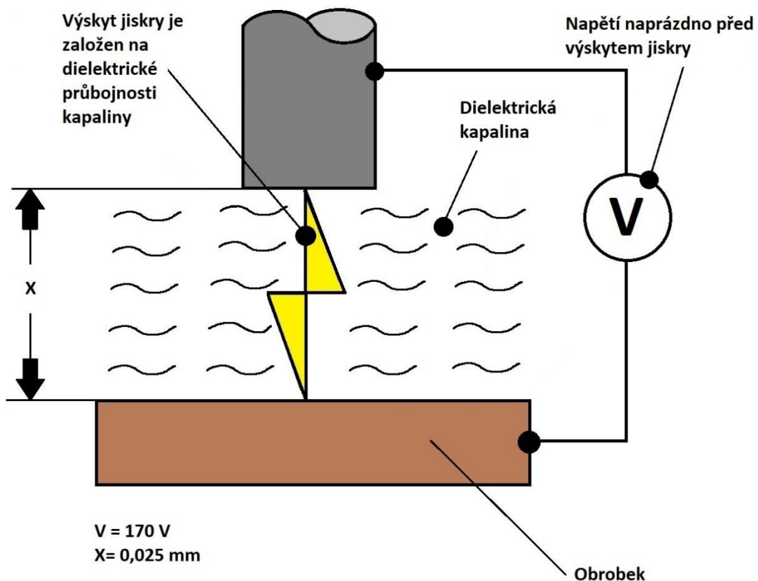
Obr. 2.11 Dielektrická průbojnost [8].
