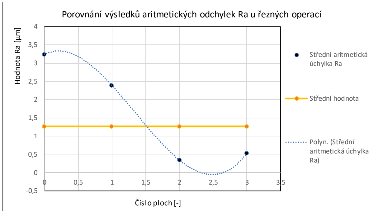
Obr. 4.18 Závislost řezných ploch na aritmetické úchlce Ra .
