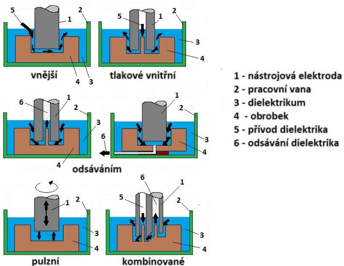
Obr. 2.21 Způsoby vyplachování [15].
