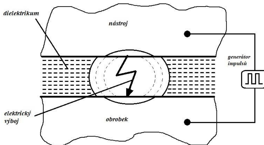
Obr. 2.5 Princip elektroeroze [7].
