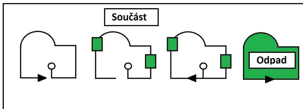
Obr. 3.14 Řezání matic [2].
