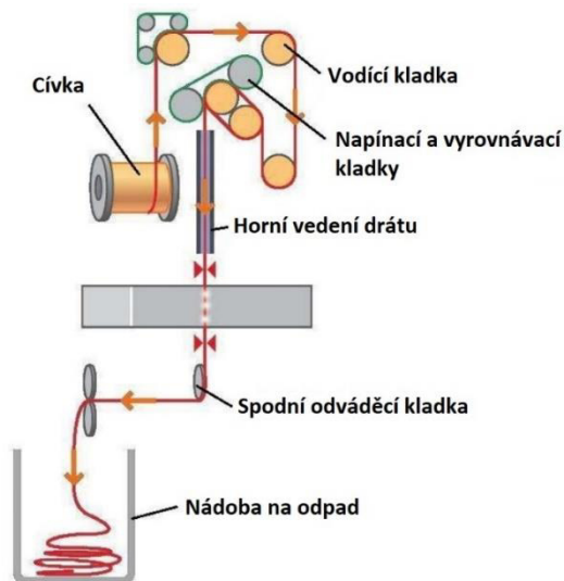
Obr. 3.9 Vedení drátu [29].
