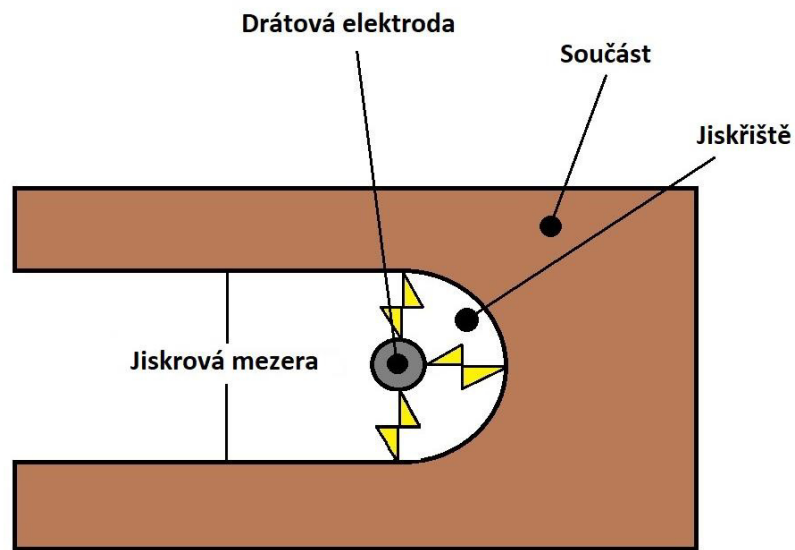
Obr. 2.2 Elektroerozivní drátové řezání (WEDM Wire Electrical Discharge Machining) [9].
