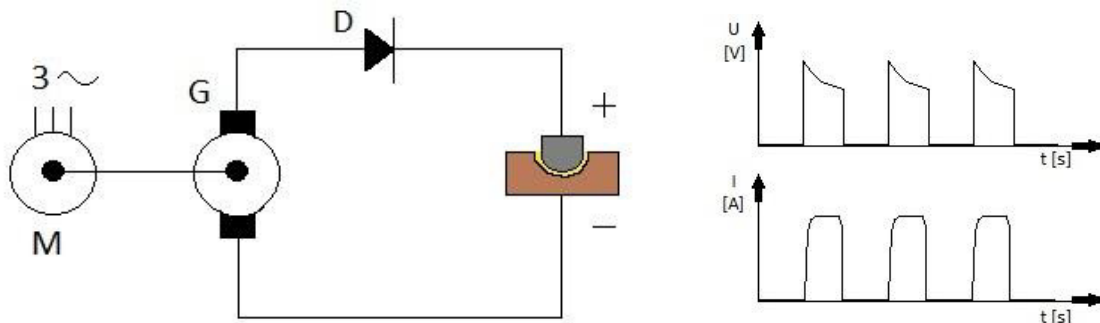
Obr. 2.15 Základní obvod rotačního generátoru a jeho časový průběh proudu I a napětí U [13].
