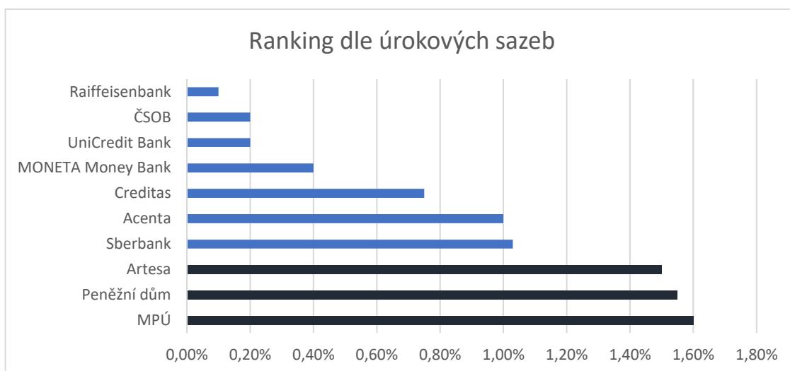
Graf 1: Ranking dle úrokových sazeb (Vlastní zpracování dle provedených analýz, 2018)
