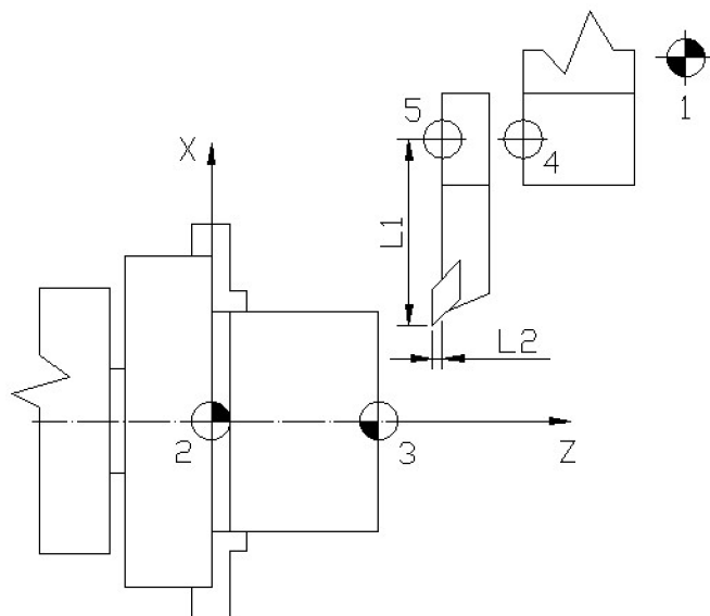
Obr. 5. Body CNC soustruhu.
