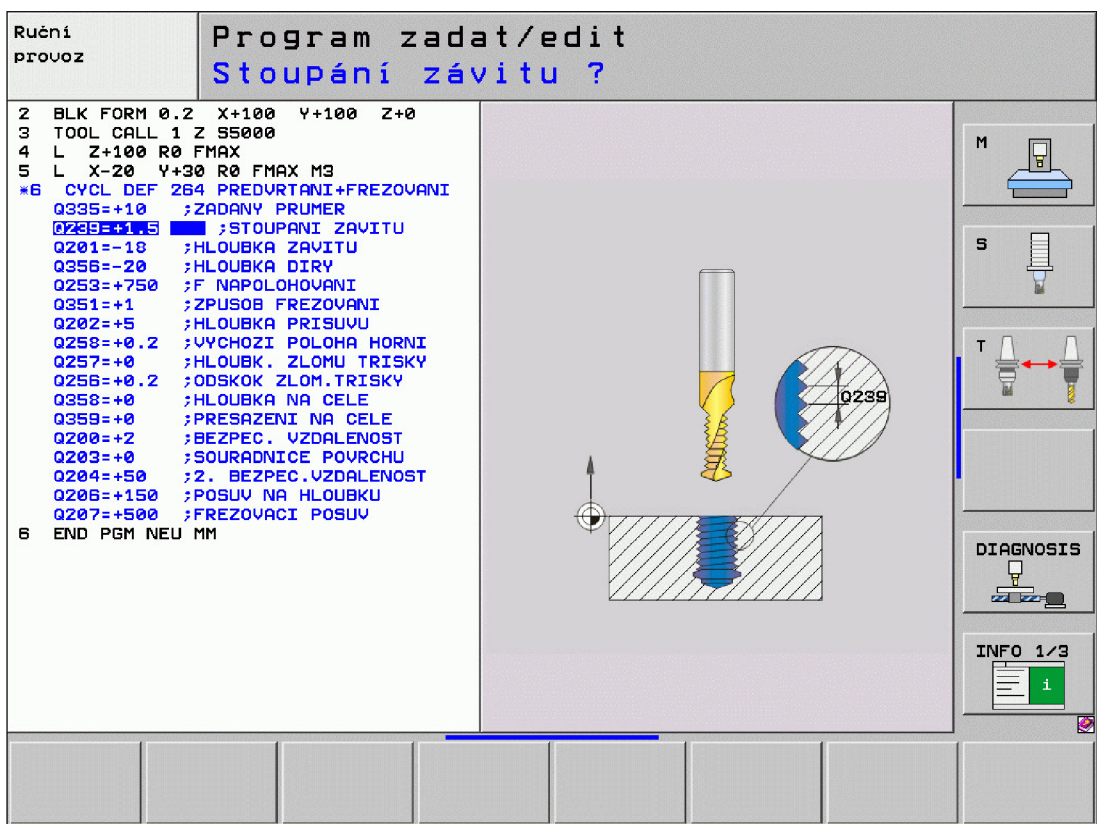
Obr. 10. Ukázka programování v popisném dialogu Heidenhain [16]
