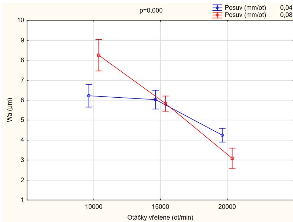
Obrázek 21: Hodnocení vlnitosti
