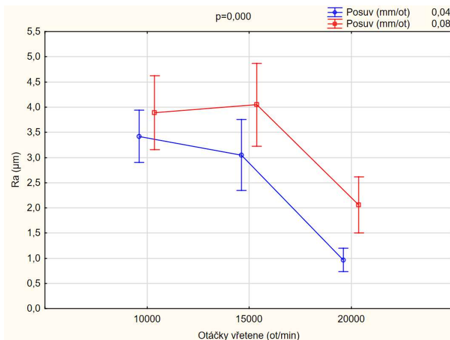
Obrázek 18: Hodnocení drsnosti
