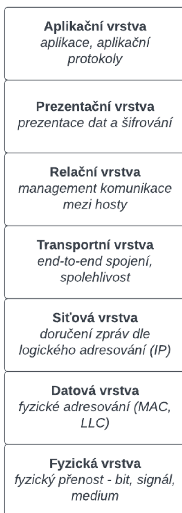
Obrázek 6: Protokolový zásobník - Referenční model ISO/OSI
