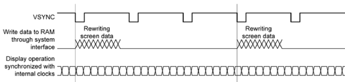
Obrázek 3.5: Přenos přes rozhraní VSYNC (převzato z [4])
