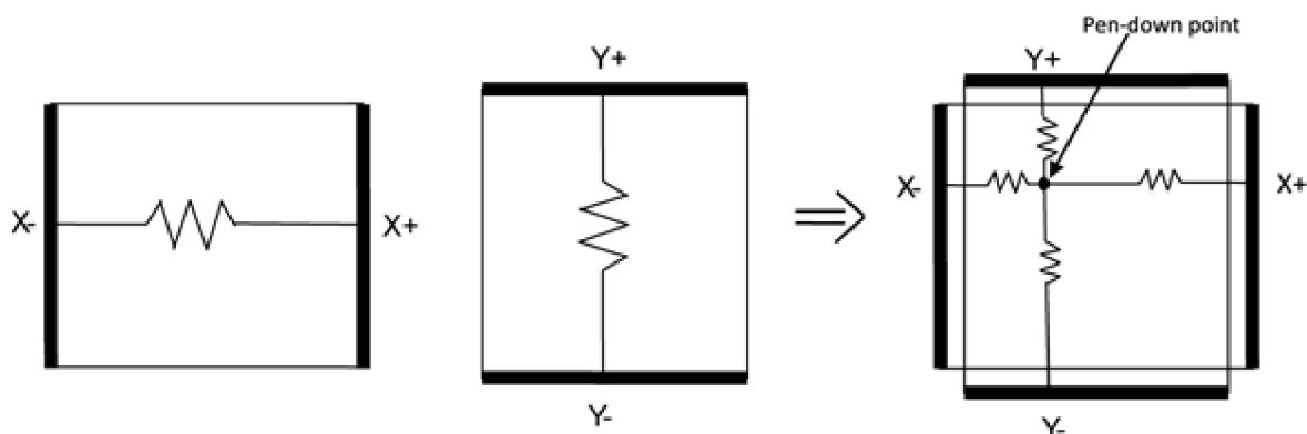
Obrázek 3.8: Schéma 4drátového dotykového displeje (převzato z [6])
