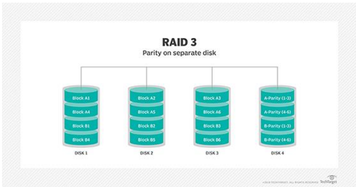
Obr. 9: RAID 3 (Zdroj: 10)
