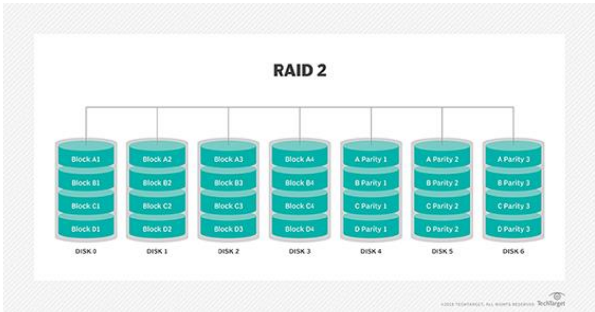
Obr. 8: RAID 2 (Zdroj: 10)
