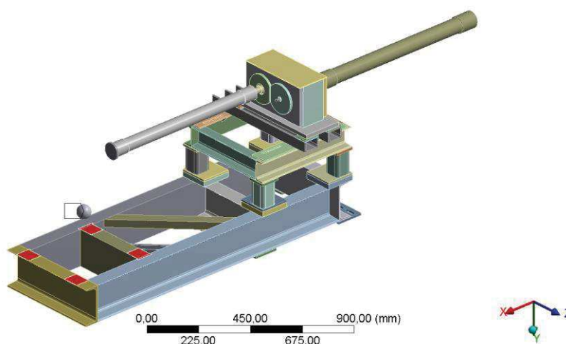
Obr. 47 Zjednodušený model v Ansys Workbench.
