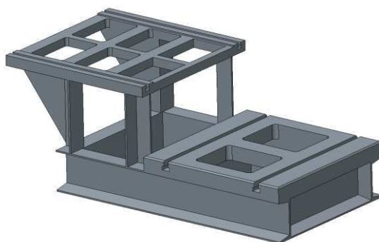
Obr. 38 Zkušební stav-svařenec (první varianta)
