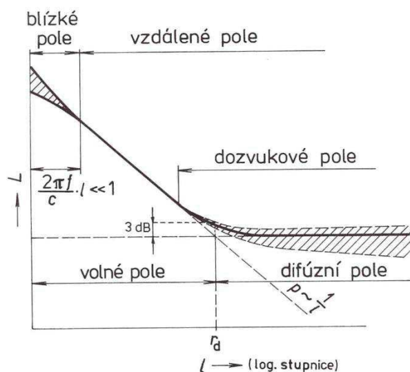
Obr. 2 Typy akustických polí[2]
