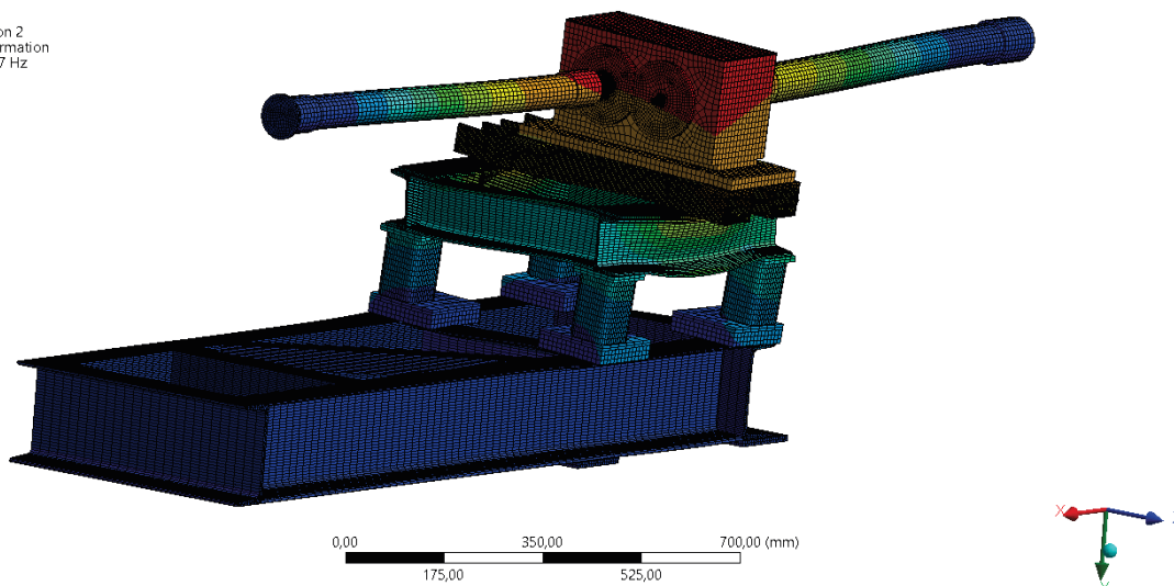
Obr. 53 Druhý vlastní tvar kmitání zkušebního stavu - 150Hz
