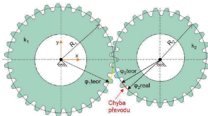
Obr. 23 Znáornění chyby převodu [8]
