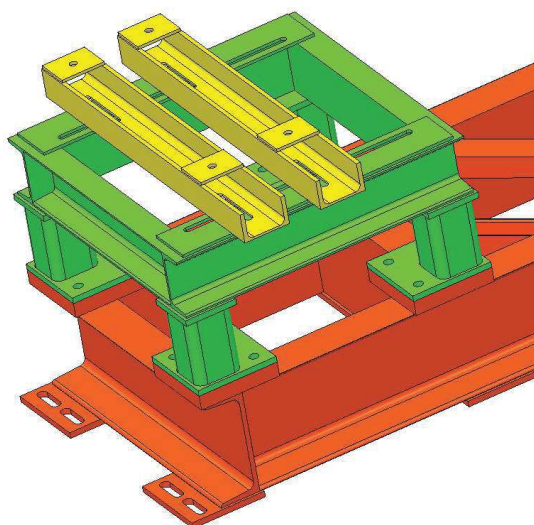
Obr. 44 Detail svařenců finálního návrhu
