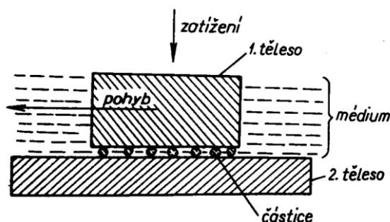
Obrázek 16 Schéma tření [7]
