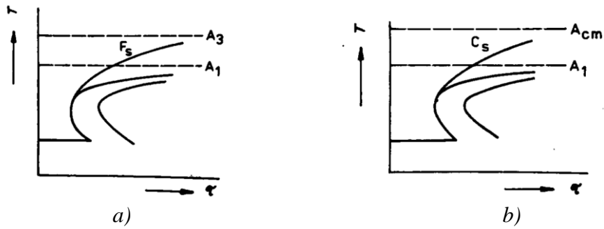
Obrázek 4 Schéma diagramu IRA pro a) podeutektoidní oceli b) nadeutektoidní oceli [2]
