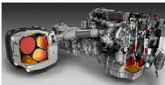
Obr. 30 Scania Euro VI [39]
