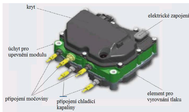
Obr. 18 Dopravní modul DNOX 2.2 [26]
