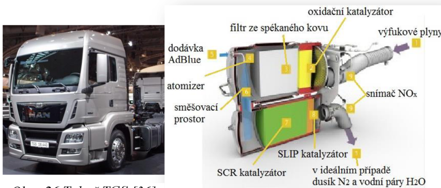
Obr. 26 Tahač TGS [36]
