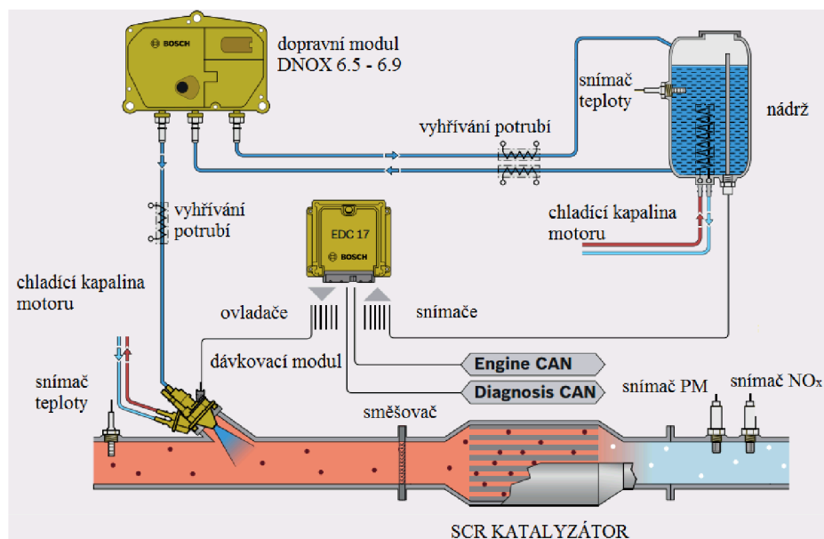
Obr. 20 Bosch denoxtronic 6.5 - 6.9 [28,29]
