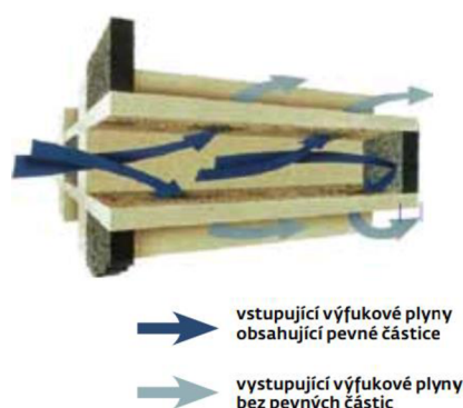
Obr. 4 Mřížka DPF [50]
