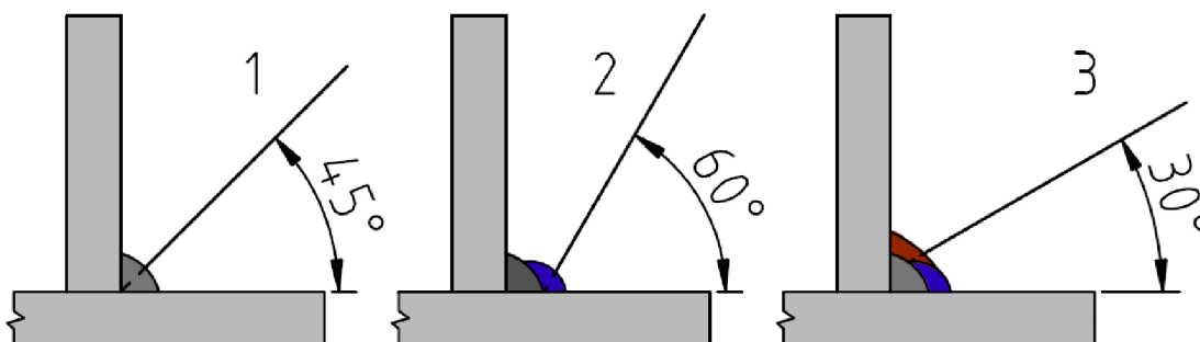
Obr. 59 Doporučený sklon elektrody pro třívrstvý svarový spoj FW PB. [9]
