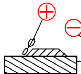
Obr. 76 Polarita nepřímá. [9]
