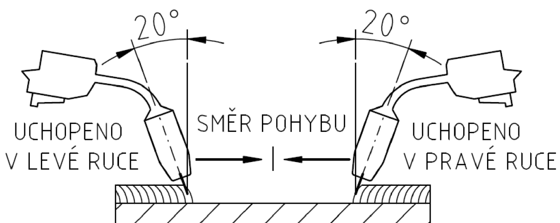
Obr. 68 Svařování vpřed. [9]
