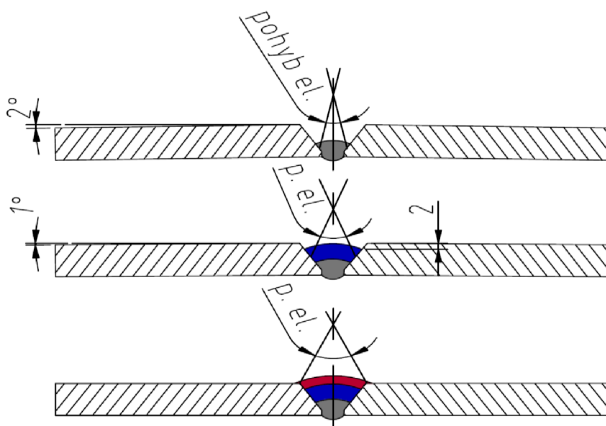
Obr. 65 Kladení jednotlivých vrstev s dráhou pohybu elektrody. [9]
