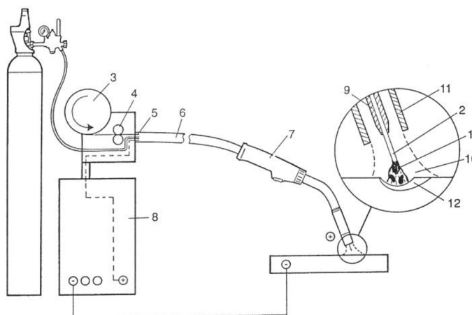
Obr. 56 Základní schéma svařovacího zařízení MIG/MAG. [12]
